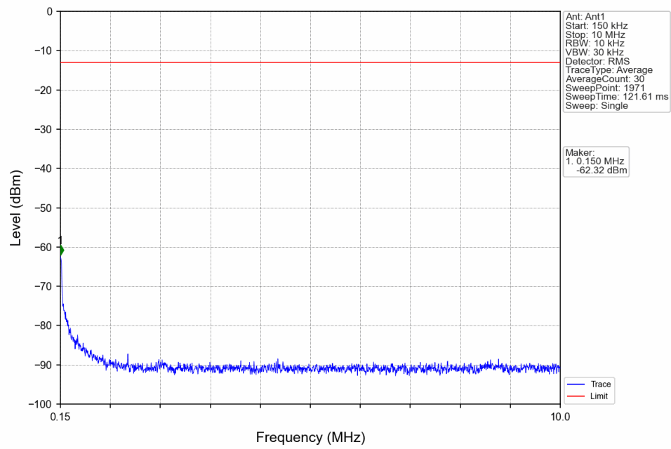
Band5_5MHz_QPSK_HCH_846.5MHz_RB_1_24_NTNV
