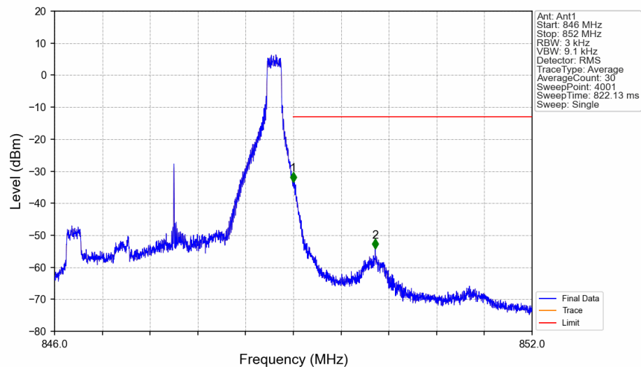
Band5_3MHz_QPSK_HCH_847.5MHz_RB_1_14_NTNV
