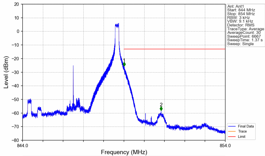
Band5_5MHz_QPSK_HCH_846.5MHz_RB_1_24_NTNV
