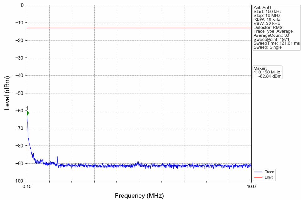
Band5_3MHz_QPSK_HCH_847.5MHz_RB_1_14_NTNV
