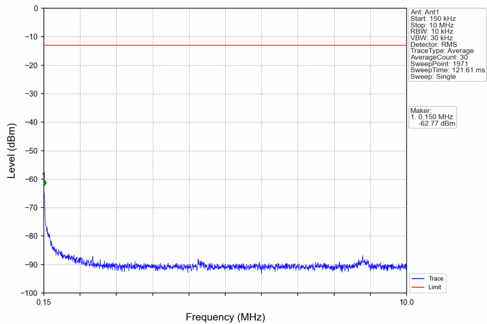
Band5_10MHz_QPSK_HCH_844MHz_RB_1_49_NTNV
