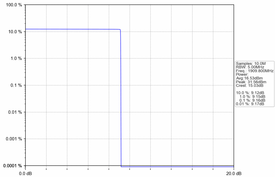
PCS1900_GSM_HCH_1909.8MHz_GSM_NTNV
