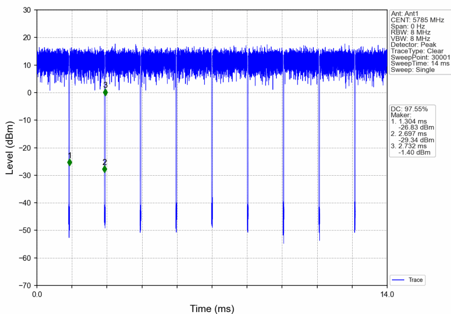
802.11a_MCH_5785MHz_Ant1_NTNV
