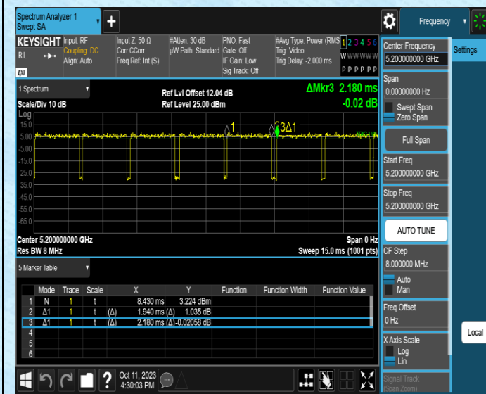
NTNV-11AC20MIMO-Ant1-5200
