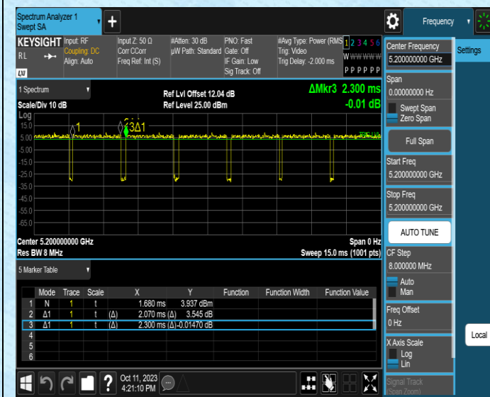
NTNV-11N20MIMO-Ant1-5200
