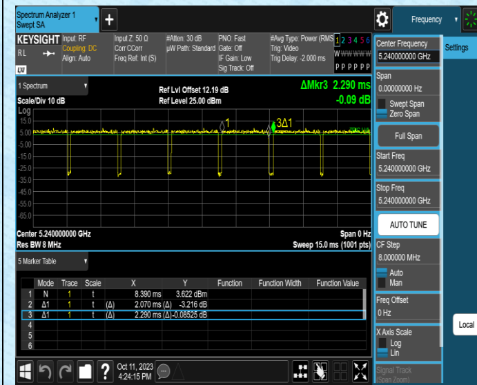
NTNV-11N20MIMO-Ant1-5240
