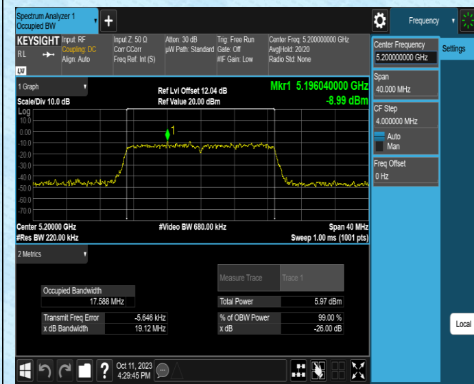
11AC20MIMO-Ant1-5200
