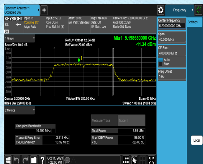
11N20MIMO-Ant2-5200
