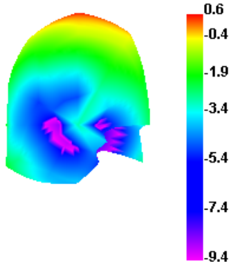
2450.000MHz E1
