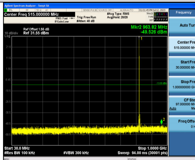
GPRS850-128-30~1000MHz
