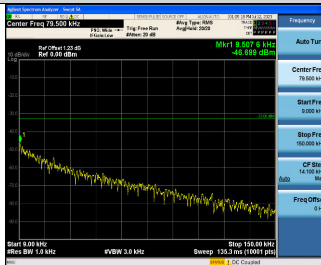
GSM850-190-0.009~0.15MHz
