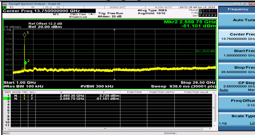
11B_Ant1_2462_1000~26500
