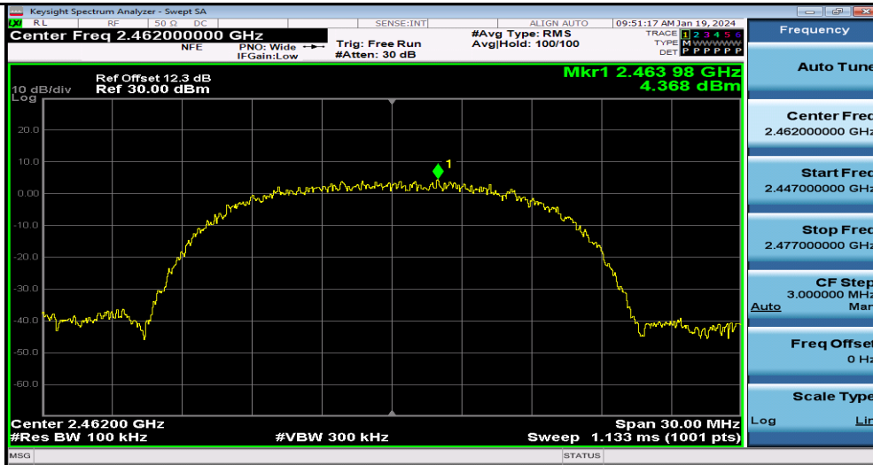
11B_Ant1_2462_0~Reference
