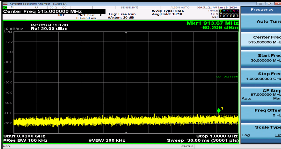
11B_Ant1_2462_30~1000
