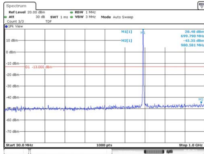
Band12-1.4MHz-QPSK-23017-1RB#0-Range1:30~1000MHz
