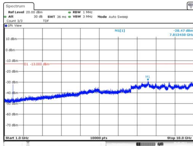
Band12-1.4MHz-QPSK-23017-1RB#0-Range2:1000~10000MHz
