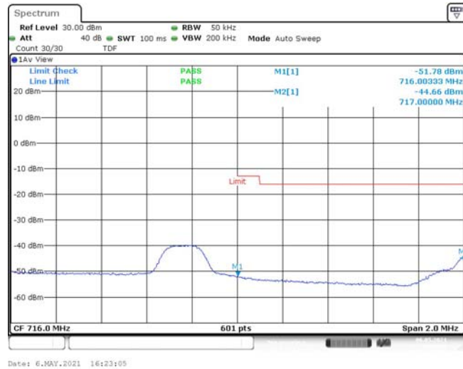
Band12-3MHz-QPSK-23165-1RB#14
