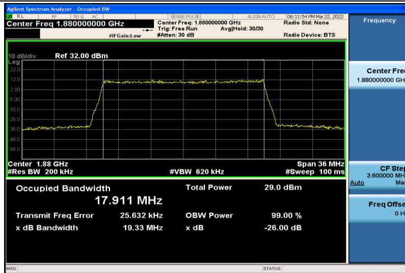
Band2-20MHz-QPSK-18900-100RB#0-17.911
