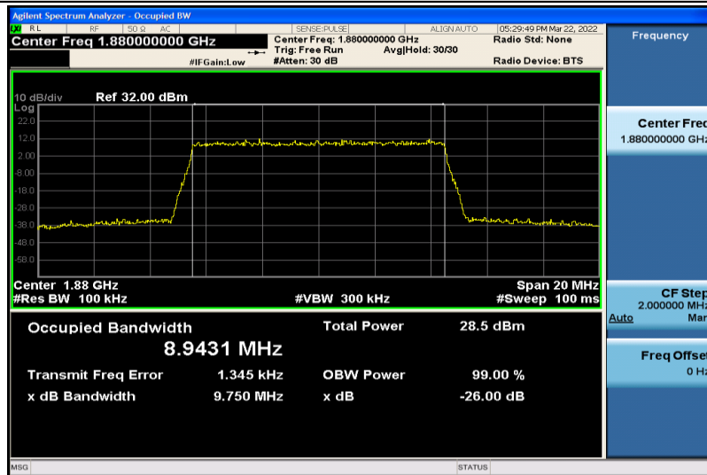
Band2-10MHz-QPSK-18900-50RB#0-8.9431
