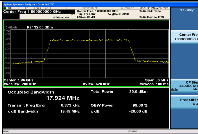
Band2-20MHz-QPSK-18700-100RB#0-17.924
