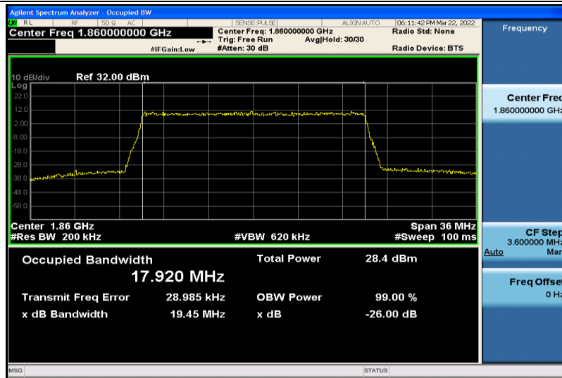
Band2-20MHz-16QAM-18700-100RB#0-17.920
