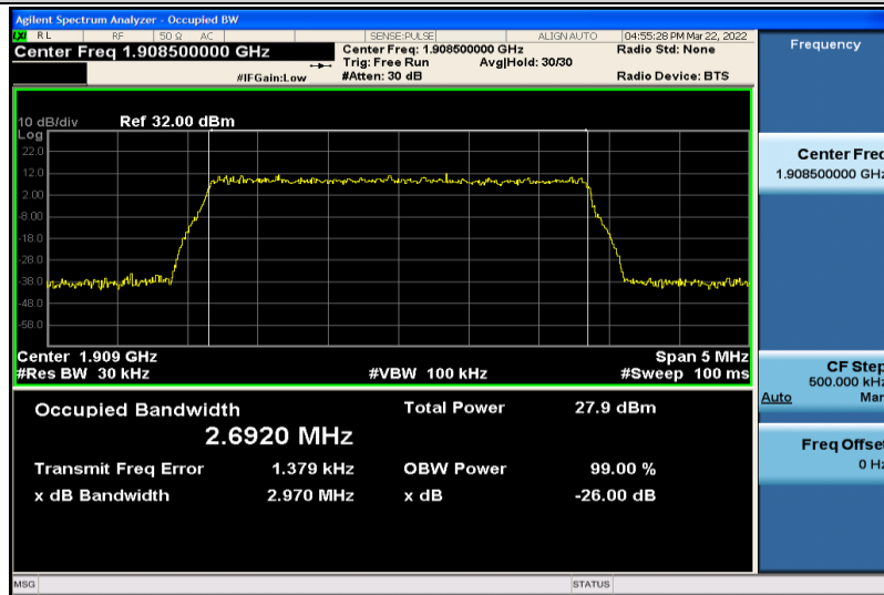
Band2-3MHz-QPSK-19185-15RB#0-2.6920
