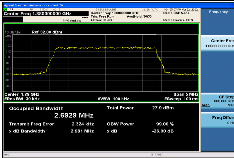
Band2-3MHz-QPSK-18900-15RB#0-2.6929
