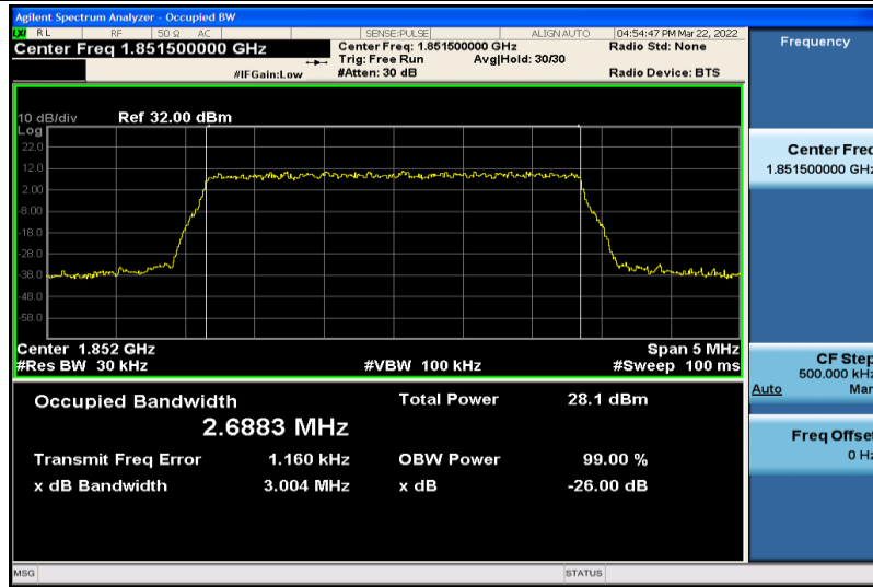
Band2-3MHz-QPSK-18615-15RB#0-2.6883
