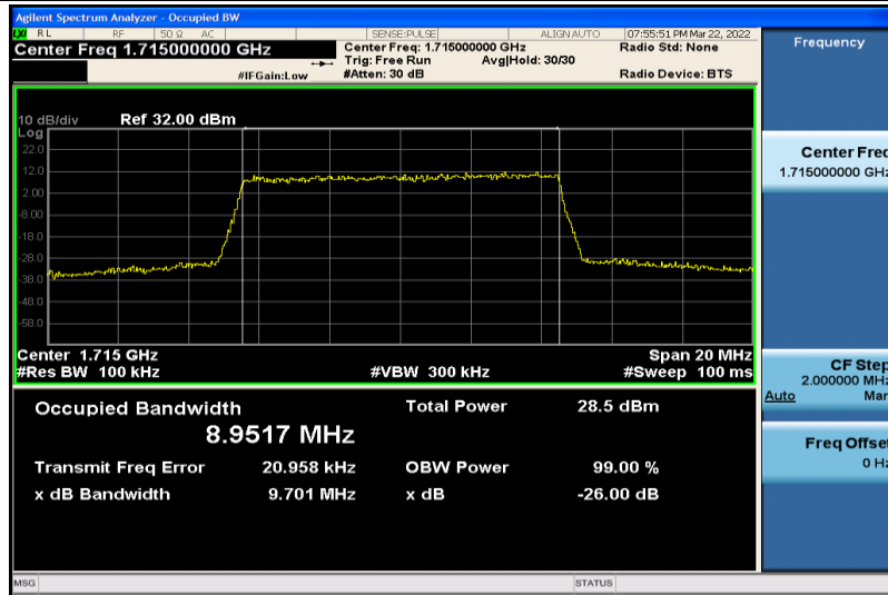
Band4-10MHz-QPSK-20000-50RB#0-8.9517
