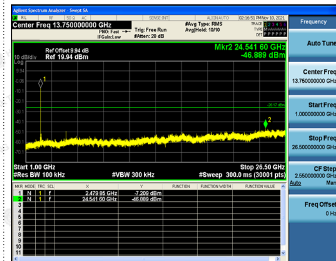
CH78
