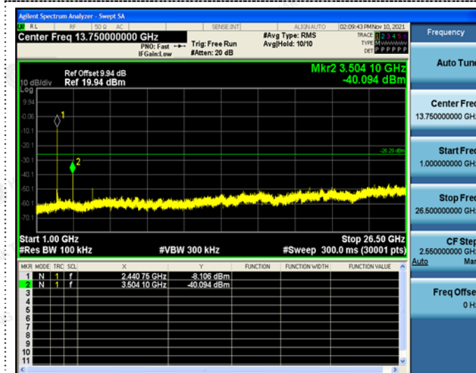
CH39
