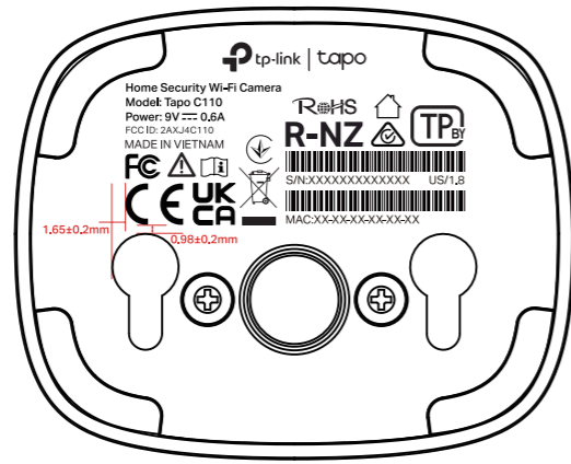
尺寸图
