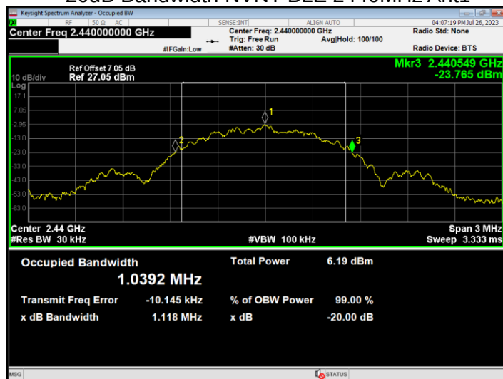
-20dB Bandwidth NVNT BLE 2440MHz Ant1
