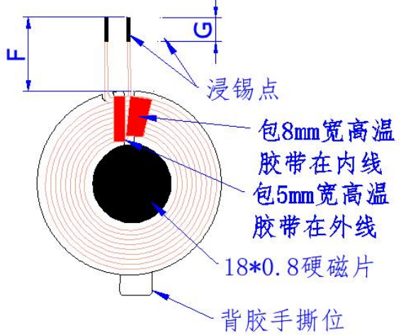
图三、线圈贴合磁片模组
