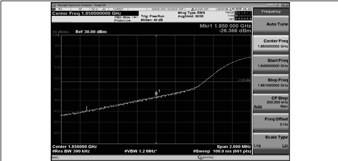
Band2-20MHz-QPSK-18700-1RB#99
