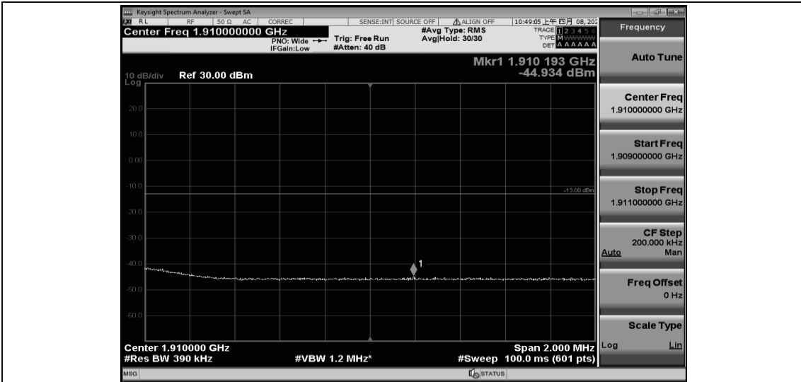
Band2-20MHz-16QAM-19100-1RB#99
