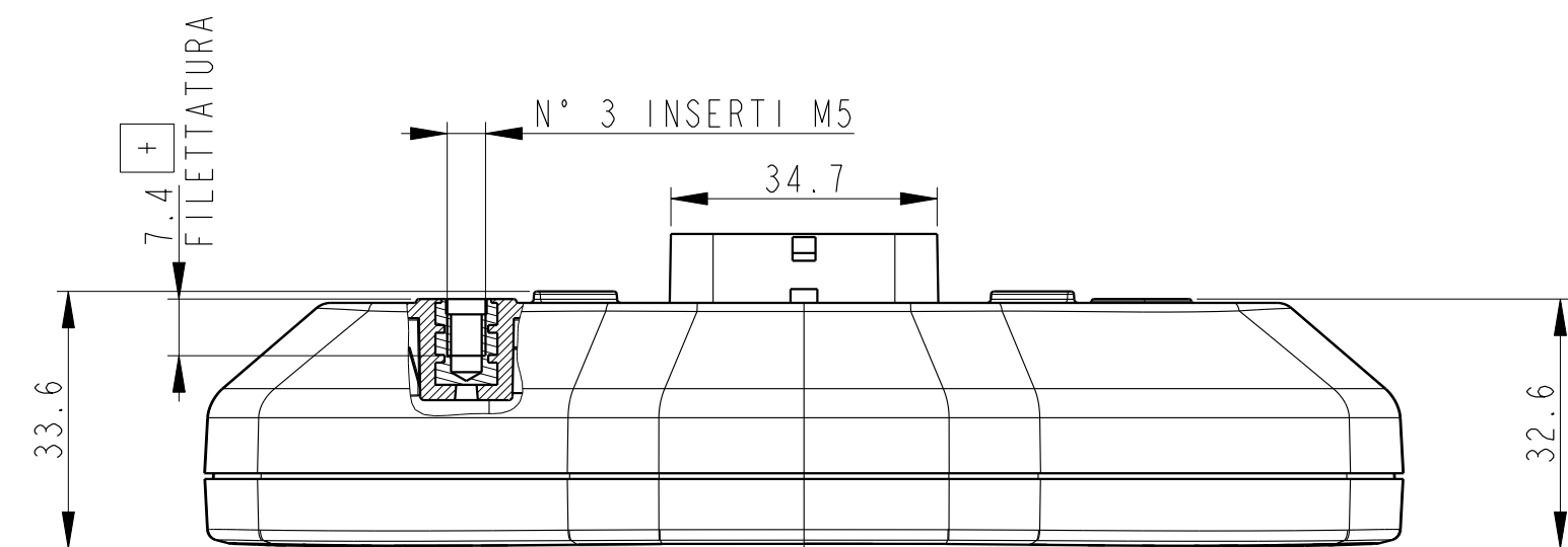
SEZIONE B-B
