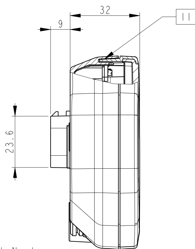
SEZIONE E-E
