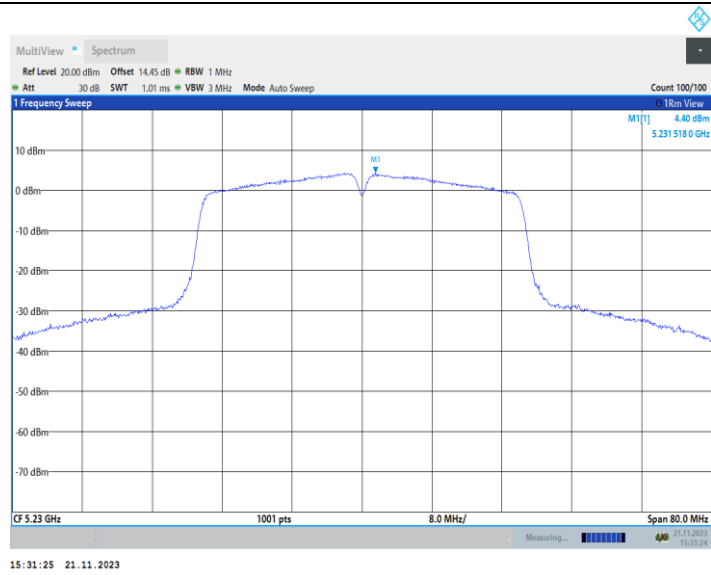
11AC40MIMO_Ant2_5230
