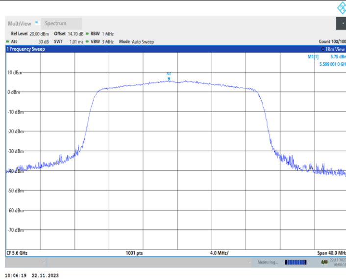
11AX20MIMO_Ant2_5600
