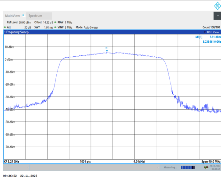
11AX20MIMO_Ant2_5240
