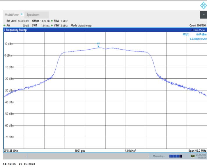
11AC20MIMO_Ant2_5280
