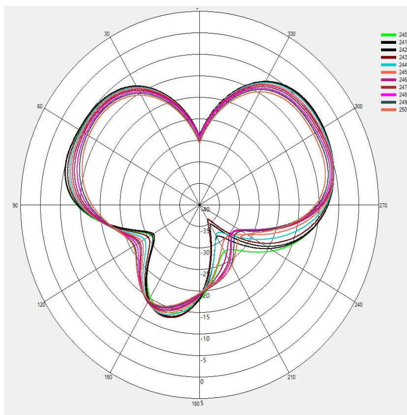
(3) Y-Z Plane(unit:dBi):
