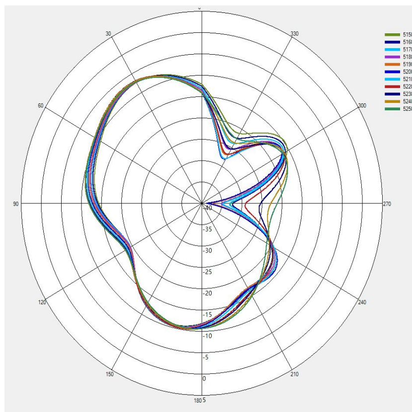
(5) X-Y Plane(unit:dBi)
