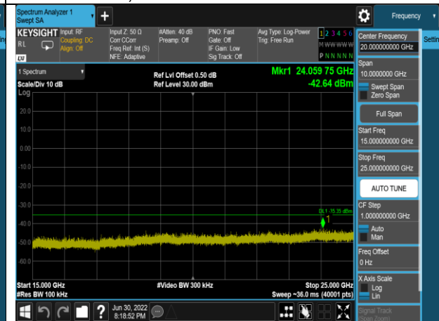
802.11n(HT40),2452MHz,Ant0,Plot 6,15000MHz~25000MHz
