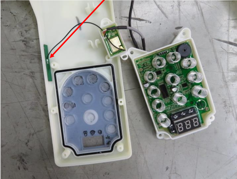
Antenna
