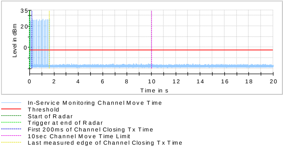
IEEE 802.11a 5700MHz
