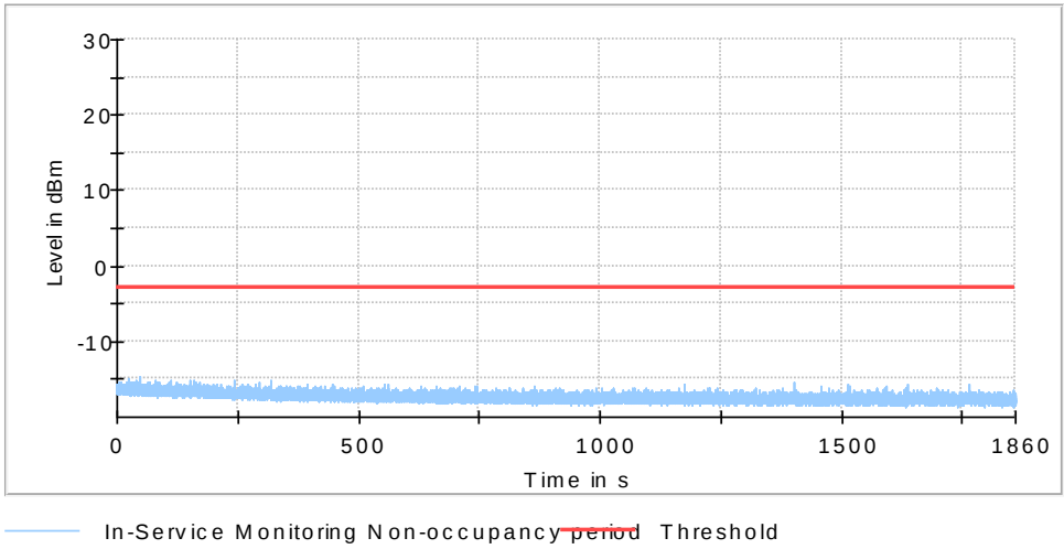
IEEE 802.11a 5700MHz
