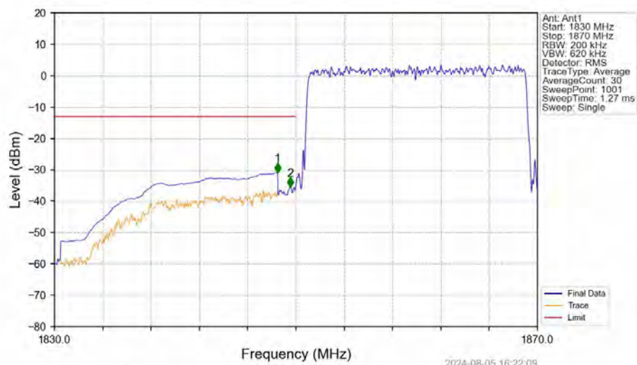
Band25_20MHz_QPSK_LCH_1860MHz_RB_100_0_NTNV
