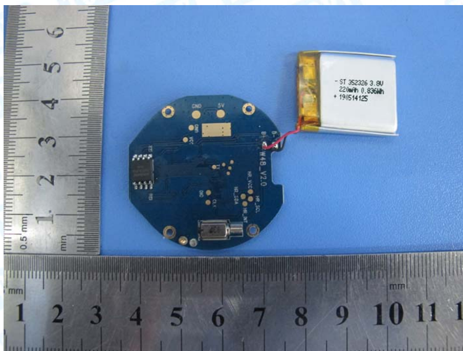
Photo 11 Battery Parameter
