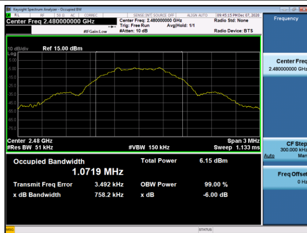
BLE 1M (CH39 : 2480 MHz) : 99% OBW
