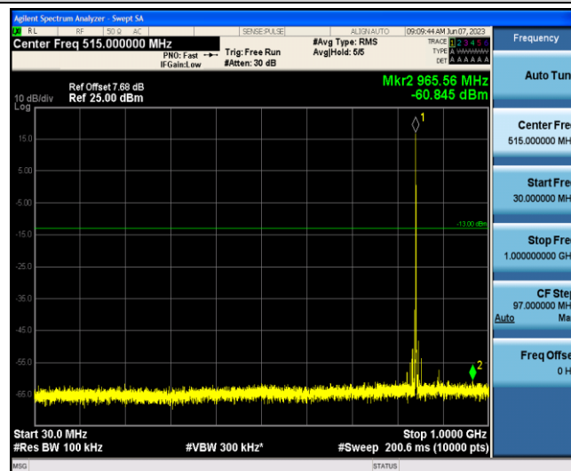
Band5-5MHz-QPSK-20625-1-0-Low-30-1000--60.85-PASS
