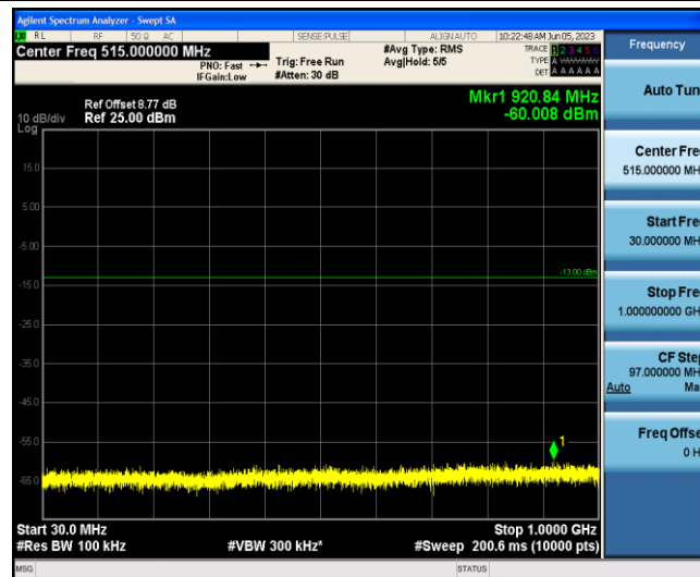
Band4-15MHz-QPSK-20025-1-0-Low-30-1000--60.01-PASS
