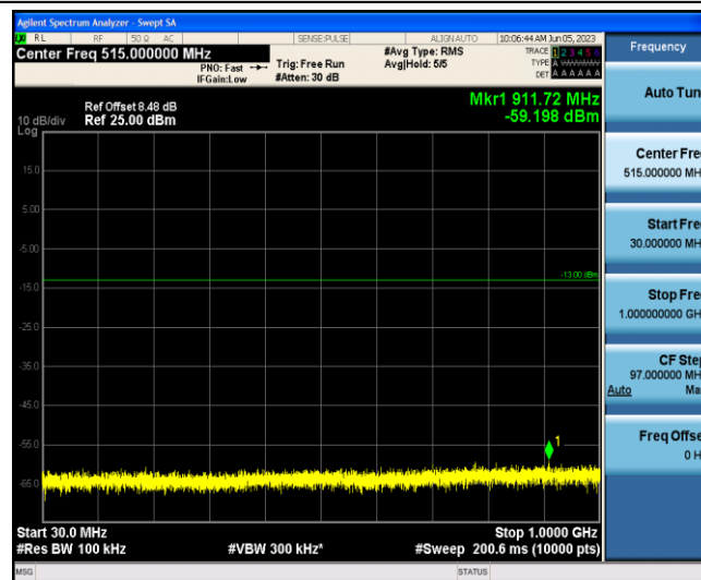
Band4-10MHz-16QAM-20350-1-0-Low-30-1000--59.2-PASS
