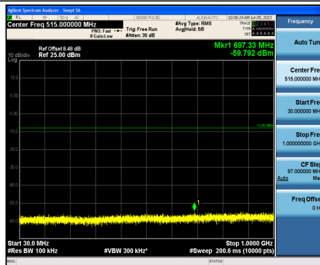
Band4-10MHz-QPSK-20350-1-0-Low-30-1000--59.79-PASS
