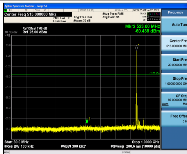
Band5-3MHz-16QAM-20635-1-0-Low-30-1000--60.44-PASS
