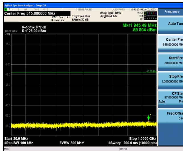
Band4-20MHz-QPSK-20050-1-0-Low-30-1000--59.8-PASS
