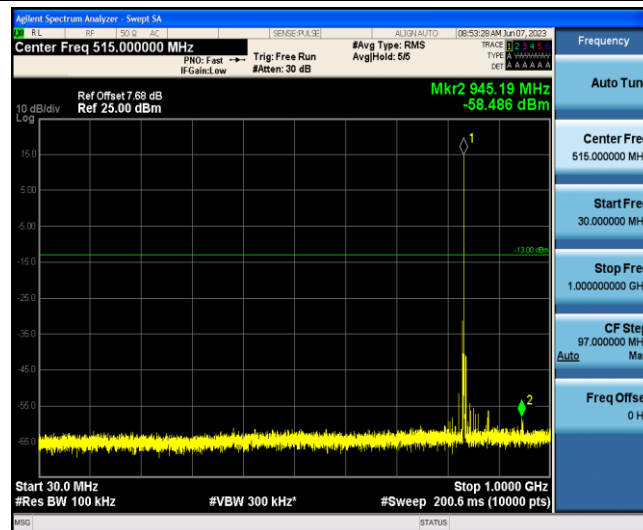
Band5-3MHz-16QAM-20525-1-0-Low-30-1000--58.49-PASS
