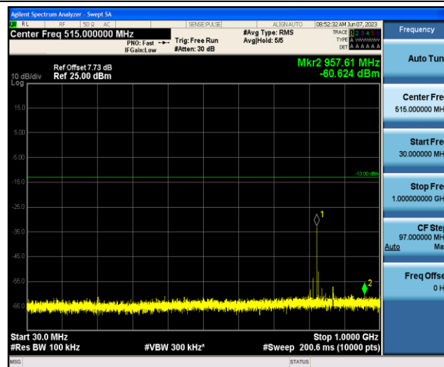
Band5-3MHz-QPSK-20415-1-0-Low-30-1000--60.62-PASS
