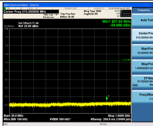
Band4-20MHz-16QAM-20050-1-0-Low-30-1000--59.69-PASS
