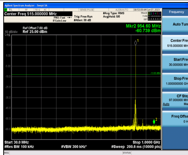
Band5-3MHz-QPSK-20525-1-0-Low-30-1000--60.74-PASS
