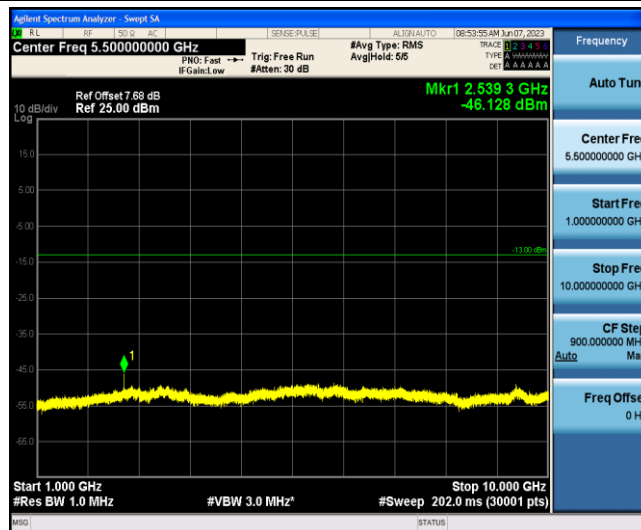
Band5-3MHz-QPSK-20635-1-0-Low-1000-10000--46.13-PASS
