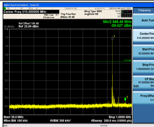
Band5-3MHz-QPSK-20635-1-0-Low-30-1000--59.43-PASS
