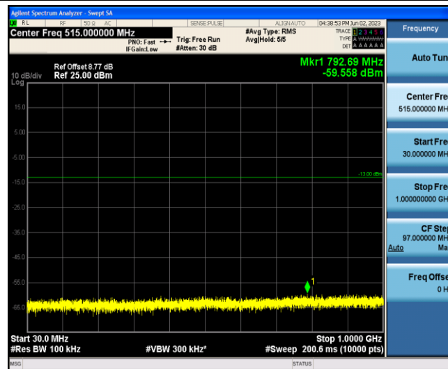
Band4-3MHz-QPSK-19965-1-0-Low-30-1000--59.56-PASS
