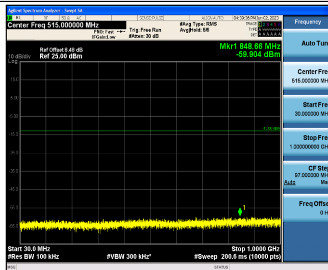
Band4-3MHz-QPSK-20175-1-0-Low-30-1000--59.9-PASS
