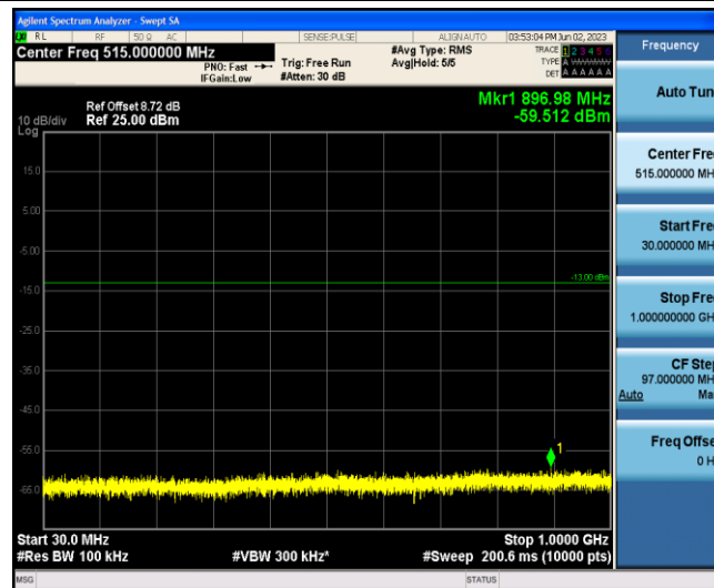
Band2-20MHz-QPSK-18700-1-0-Low-30-1000--59.51-PASS
