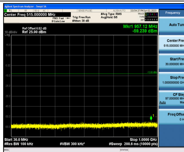
Band2-20MHz-QPSK-19100-1-0-Low-30-1000--59.24-PASS
