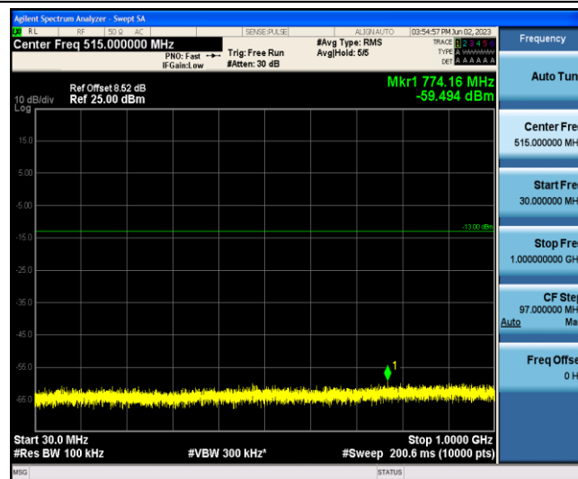
Band2-20MHz-16QAM-19100-1-0-Low-30-1000--59.49-PASS
