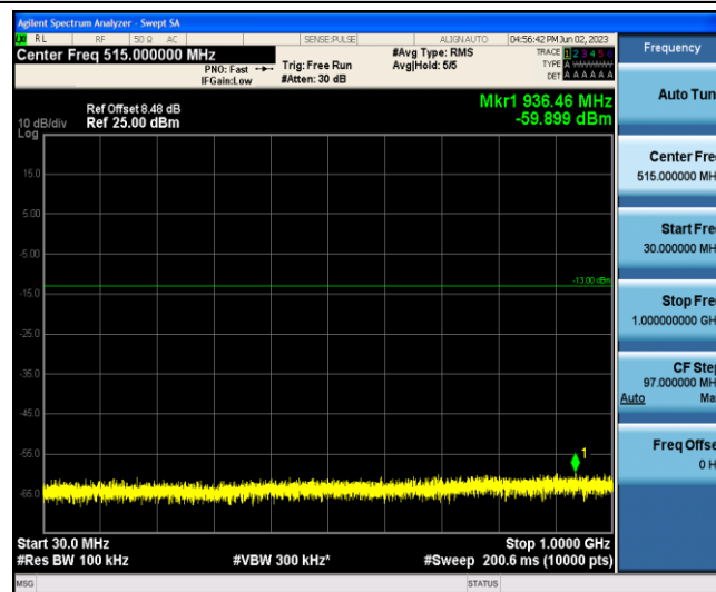
Band4-5MHz-QPSK-20375-1-0-Low-30-1000--59.9-PASS
