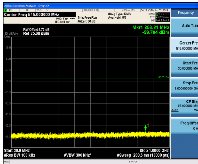
Band4-1.4MHz-16QAM-19957-1-0-Low-30-1000--59.7-PASS
