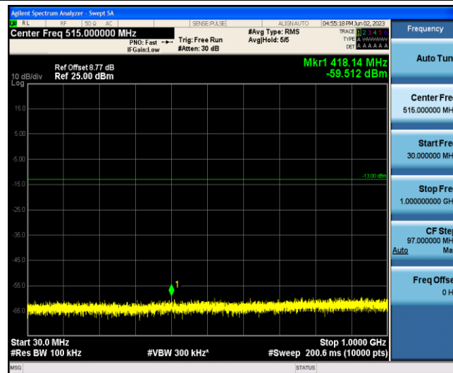
Band4-5MHz-QPSK-19975-1-0-Low-30-1000--59.51-PASS
