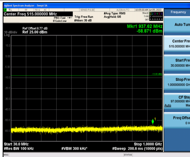
Band4-10MHz-QPSK-20000-1-0-Low-30-1000--58.87-PASS
