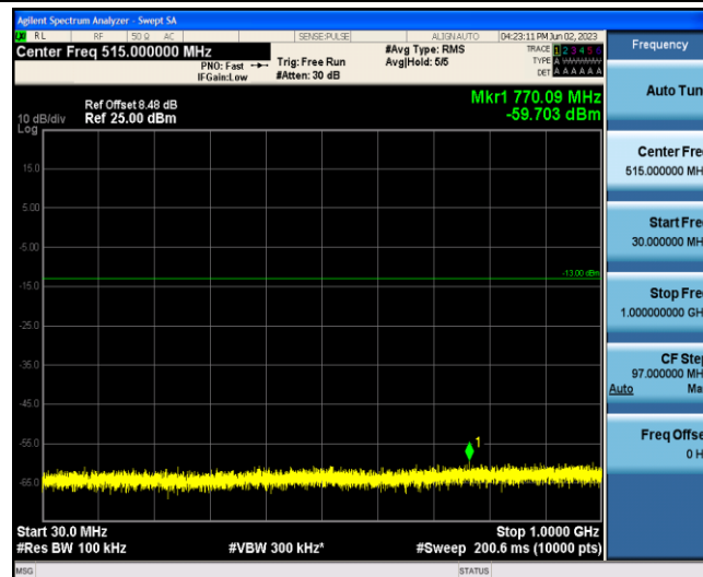
Band4-1.4MHz-QPSK-20175-1-0-Low-30-1000--59.7-PASS
