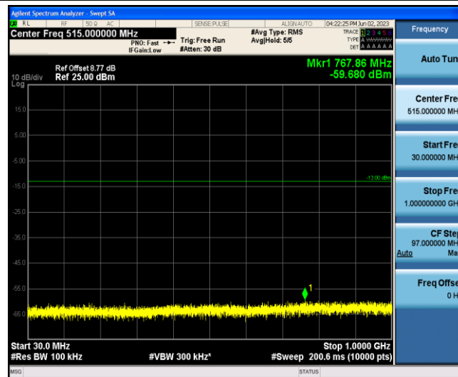
Band4-1.4MHz-QPSK-19957-1-0-Low-30-1000--59.68-PASS
