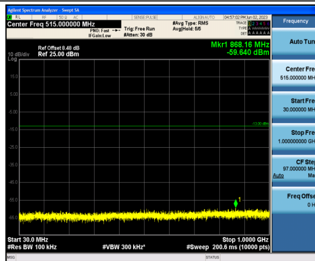
Band4-5MHz-16QAM-20375-1-0-Low-30-1000--59.64-PASS
