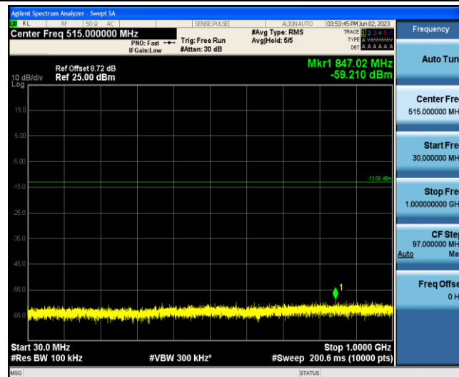
Band2-20MHz-QPSK-18900-1-0-Low-30-1000--59.21-PASS
