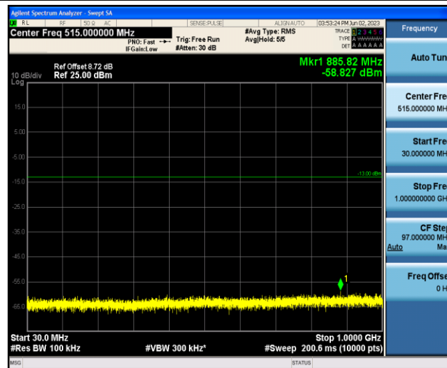
Band2-20MHz-16QAM-18700-1-0-Low-30-1000--58.83-PASS
