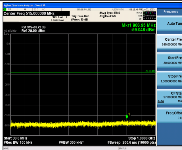
Band2-10MHz-QPSK-18900-1-0-Low-30-1000--59.05-PASS
