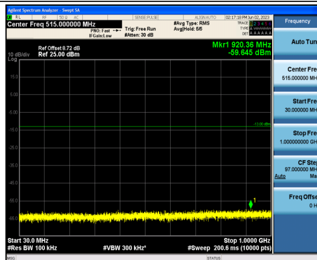
Band2-1.4MHz-16QAM-18900-1-0-Low-30-1000--59.65-PASS
