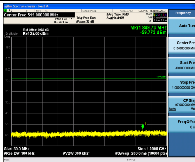
Band2-3MHz-QPSK-19185-1-0-Low-30-1000--59.77-PASS
