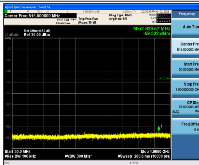
Band2-5MHz-QPSK-19175-1-0-Low-30-1000--59.52-PASS
