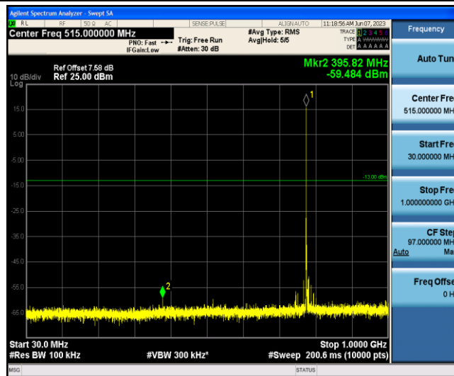
Band13-5MHz-16QAM-23230-1-0-Low-30-1000--59.48-PASS
