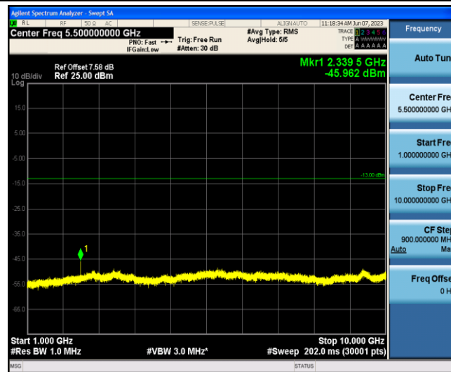
Band13-5MHz-QPSK-23230-1-0-Low-1000-10000--45.96-PASS
