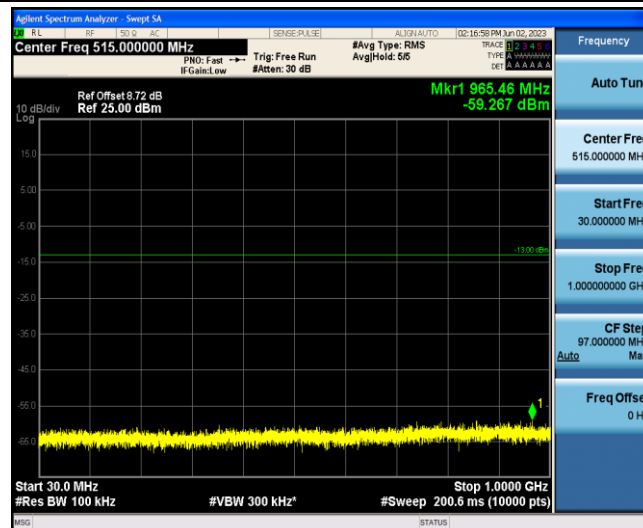
Band2-1.4MHz-QPSK-18900-1-0-Low-30-1000--59.27-PASS
