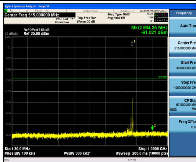
Band13-10MHz-QPSK-23230-1-0-Low-30-1000--61.02-PASS
