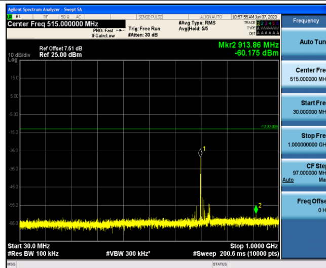
Band12-10MHz-QPSK-23095-1-0-Low-30-1000--60.18-PASS
