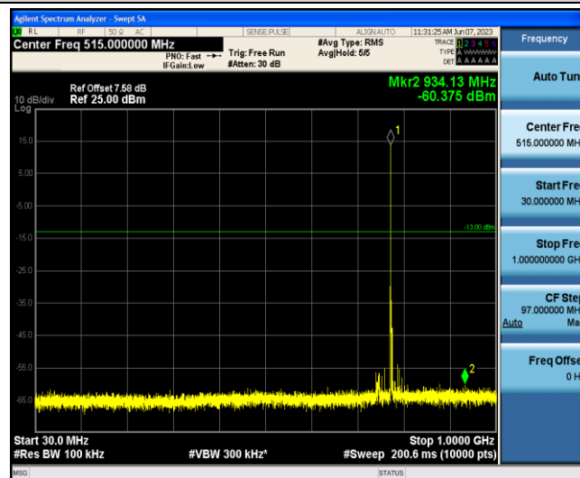
Band13-10MHz-16QAM-23230-1-0-Low-30-1000--60.38-PASS
