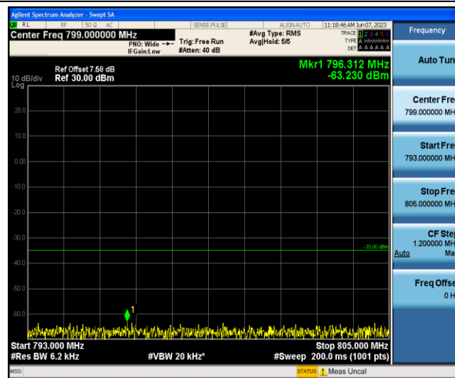
Band13-5MHz-QPSK-23230-1-0-Low-793-805--63.23-PASS
