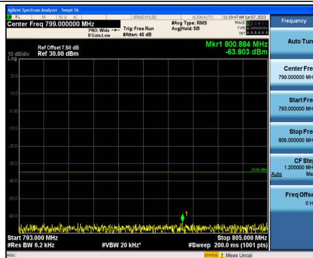
Band13-5MHz-QPSK-23255-1-0-Low-793-805--63.8-PASS
