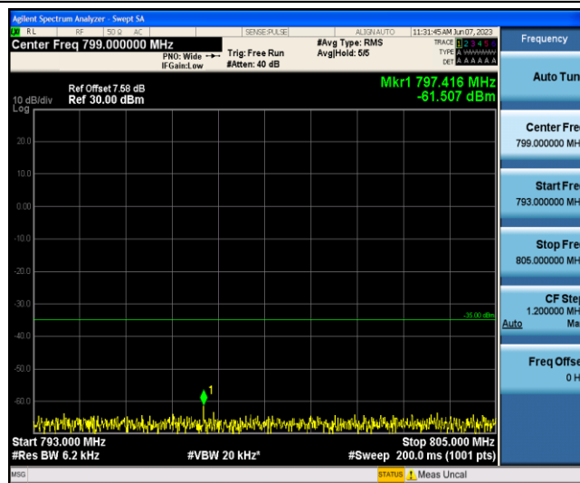
Band13-10MHz-16QAM-23230-1-0-Low-793-805--61.51-PASS
