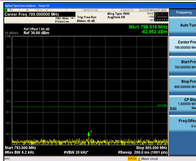
Band13-5MHz-QPSK-23205-1-0-Low-793-805--62.95-PASS
