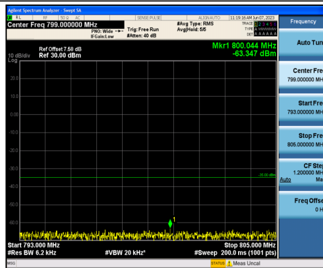
Band13-5MHz-16QAM-23230-1-0-Low-793-805--63.35-PASS
