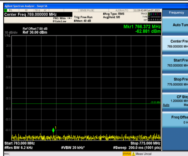
Band13-5MHz-QPSK-23255-1-0-Low-763-775--62.88-PASS
