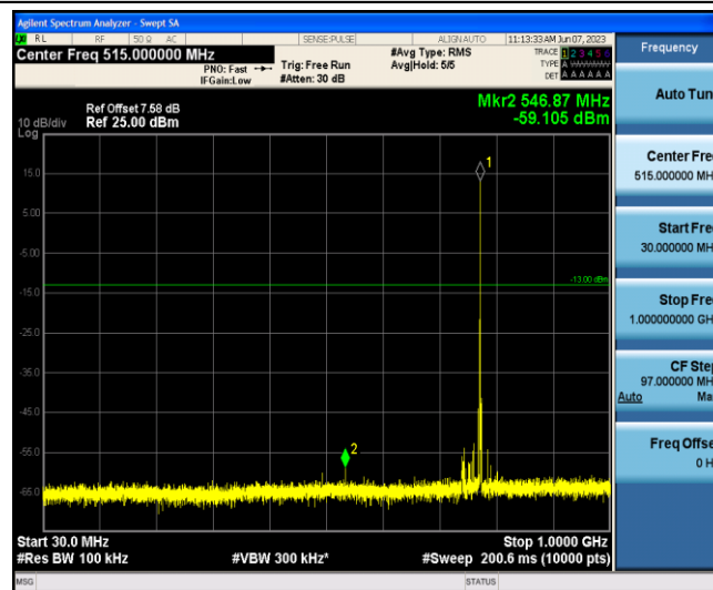
Band13-5MHz-QPSK-23205-1-0-Low-30-1000--59.11-PASS
