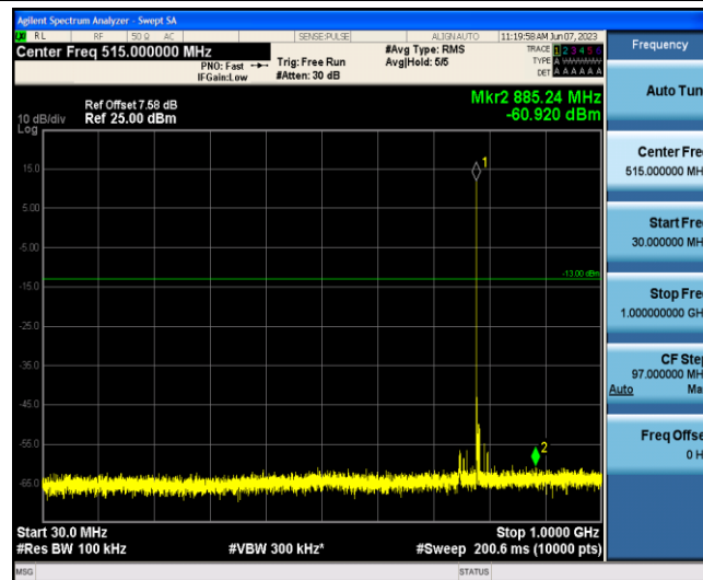
Band13-5MHz-16QAM-23255-1-0-Low-30-1000--60.92-PASS
