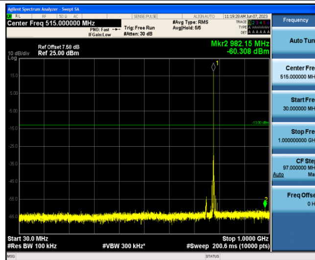
Band13-5MHz-QPSK-23255-1-0-Low-30-1000--60.31-PASS
