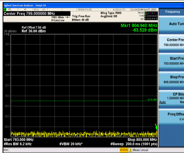
Band13-5MHz-16QAM-23205-1-0-Low-793-805--63.53-PASS
