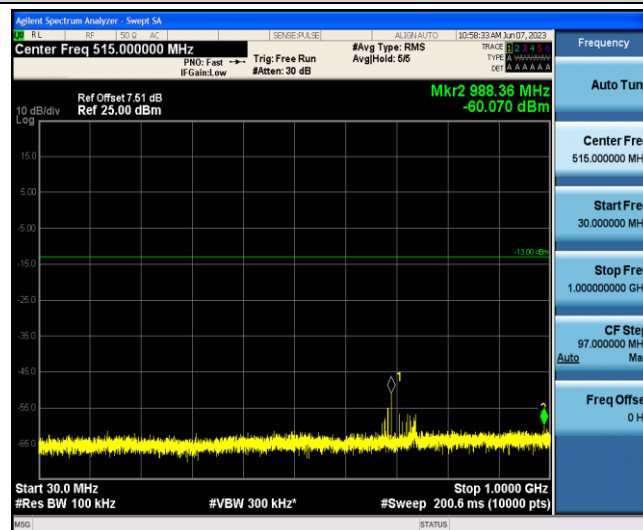
Band12-10MHz-QPSK-23130-1-0-Low-30-1000--60.07-PASS
