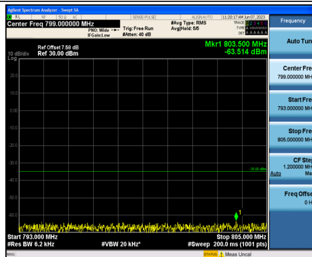
Band13-5MHz-16QAM-23255-1-0-Low-793-805--63.51-PASS
