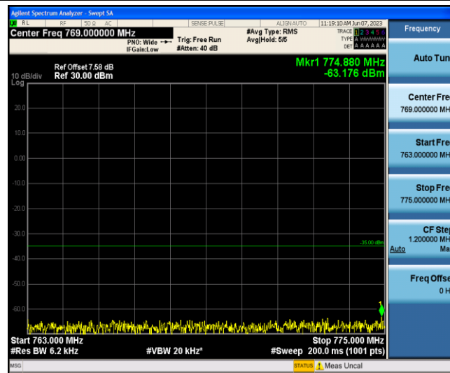
Band13-5MHz-16QAM-23230-1-0-Low-763-775--63.18-PASS
