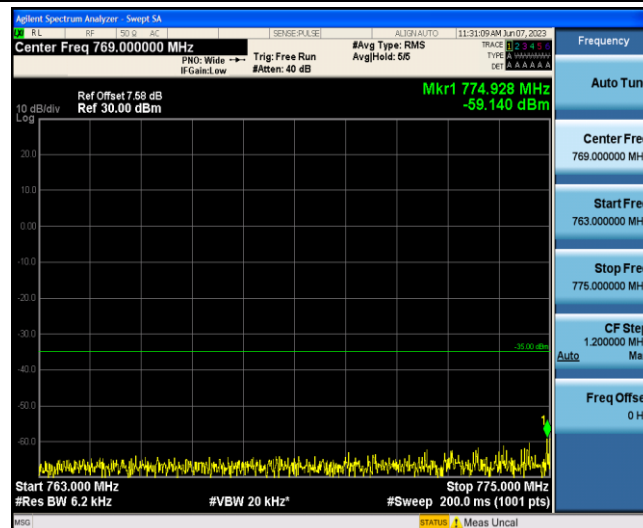
Band13-10MHz-QPSK-23230-1-0-Low-763-775--59.14-PASS
