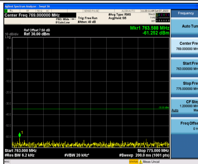
Band13-5MHz-16QAM-23255-1-0-Low-763-775--61.25-PASS
