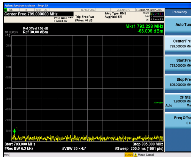
Band13-10MHz-QPSK-23230-1-0-Low-793-805--63.01-PASS
