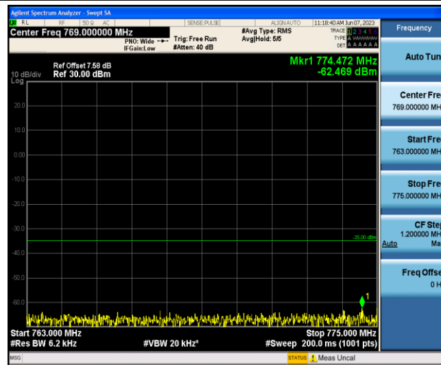
Band13-5MHz-QPSK-23230-1-0-Low-763-775--62.47-PASS
