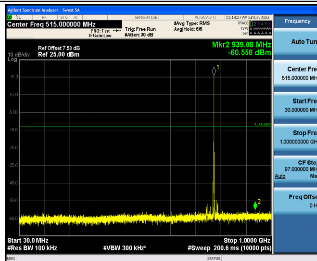
Band13-5MHz-QPSK-23230-1-0-Low-30-1000--60.56-PASS
