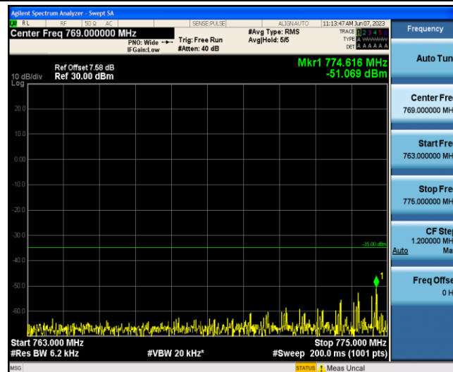
Band13-5MHz-QPSK-23205-1-0-Low-763-775--51.07-PASS
