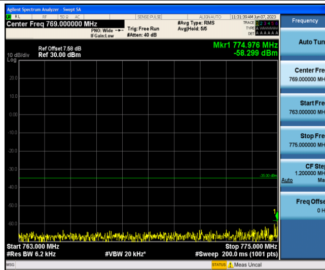
Band13-10MHz-16QAM-23230-1-0-Low-763-775--58.3-PASS
