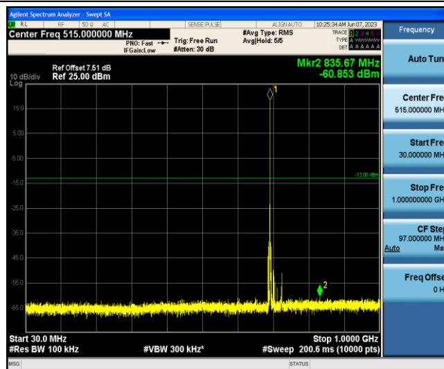
Band12-3MHz-QPSK-23025-1-0-Low-30-1000--60.85-PASS
