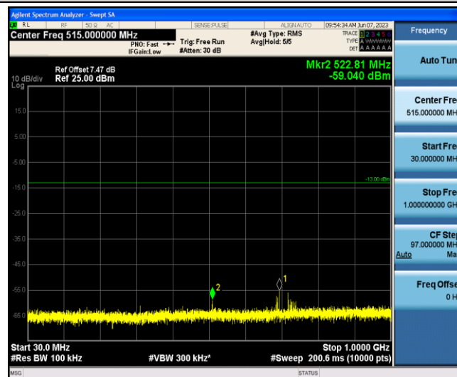
Band12-1.4MHz-QPSK-23173-1-0-Low-30-1000--59.04-PASS
