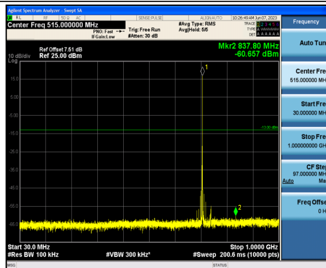
Band12-3MHz-QPSK-23165-1-0-Low-30-1000--60.66-PASS
