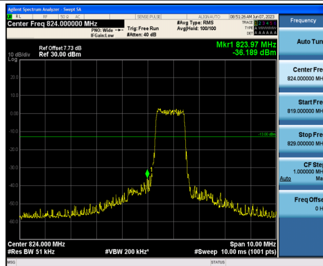
Band5-3MHz-QPSK-20415-6-0-Low--36.19-PASS
