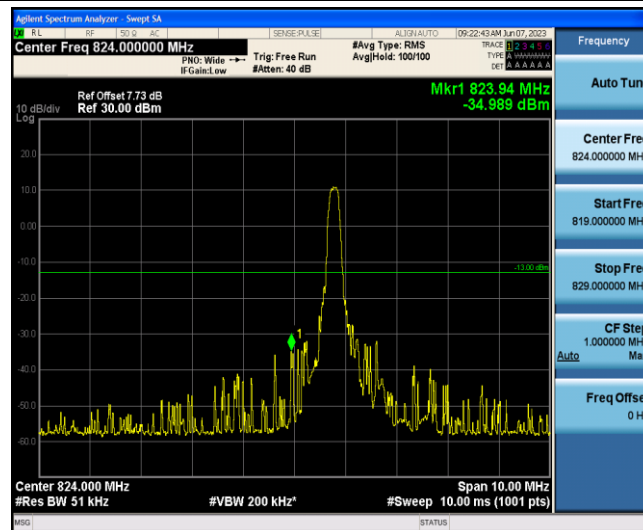
Band5-10MHz-QPSK-20450-1-0-Low--34.99-PASS
