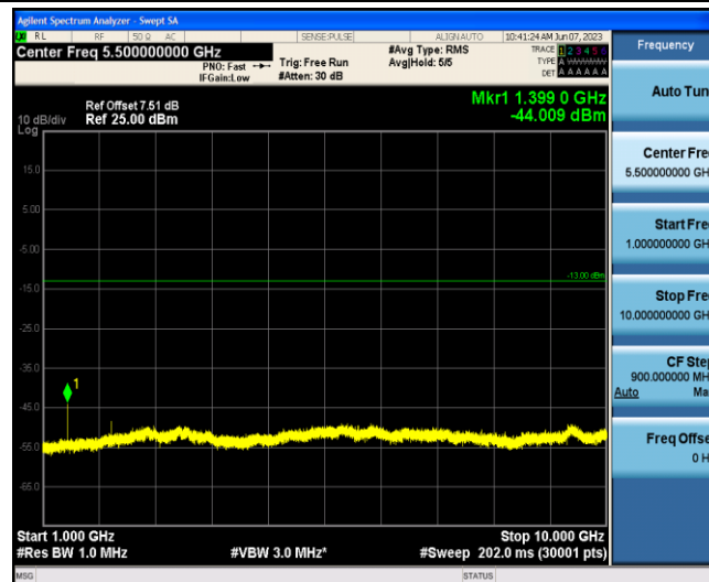
Band12-5MHz-QPSK-23035-1-0-Low-1000-10000--44.01-PASS
