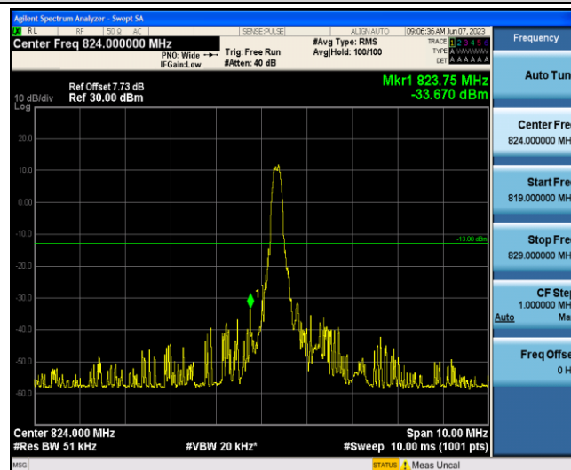
Band5-5MHz-16QAM-20425-1-0-Low--33.67-PASS
