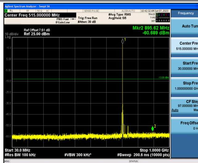
Band12-5MHz-QPSK-23155-1-0-Low-30-1000--60.69-PASS
