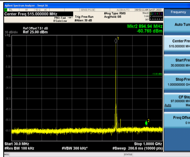
Band12-1.4MHz-QPSK-23017-1-0-Low-30-1000--60.77-PASS
