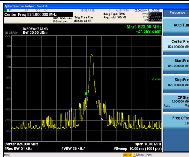
Band5-5MHz-QPSK-20425-1-0-Low--27.59-PASS
