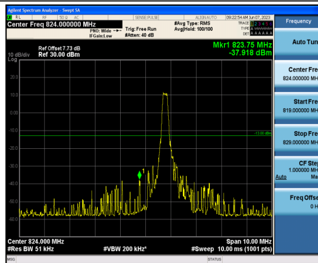
Band5-10MHz-16QAM-20450-1-0-Low--37.92-PASS
