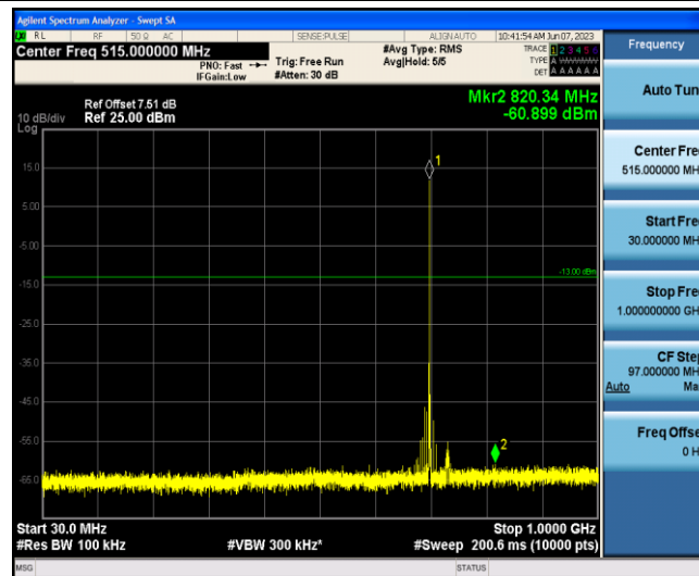
Band12-5MHz-QPSK-23095-1-0-Low-30-1000--60.9-PASS
