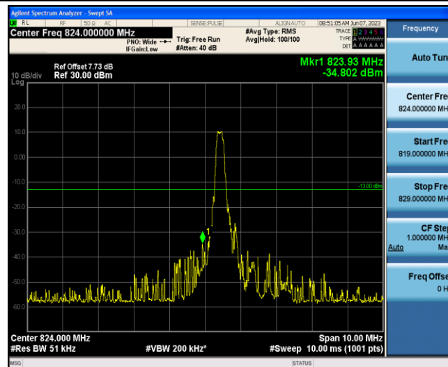
Band5-3MHz-QPSK-20415-1-0-Low--34.80-PASS
