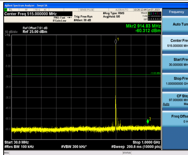
Band12-3MHz-QPSK-23095-1-0-Low-30-1000--60.31-PASS
