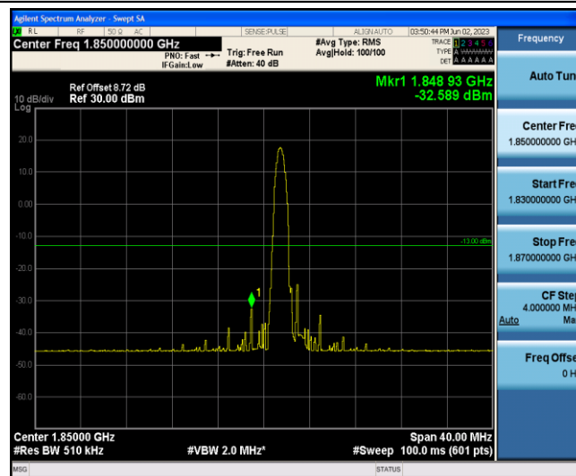
Band2-20MHz-QPSK-18700-1-0-Low--32.59-PASS
