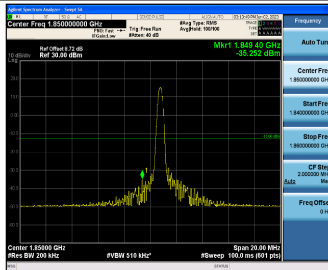
Band2-10MHz-QPSK-18650-1-0-Low--35.25-PASS
