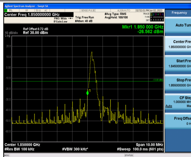
Band2-5MHz-16QAM-18625-1-0-Low--26.56-PASS
