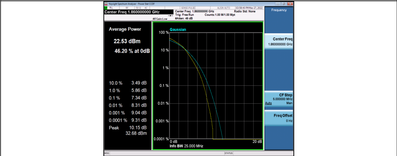
Band25-20MHz-16QAM-26365-100RB#0
