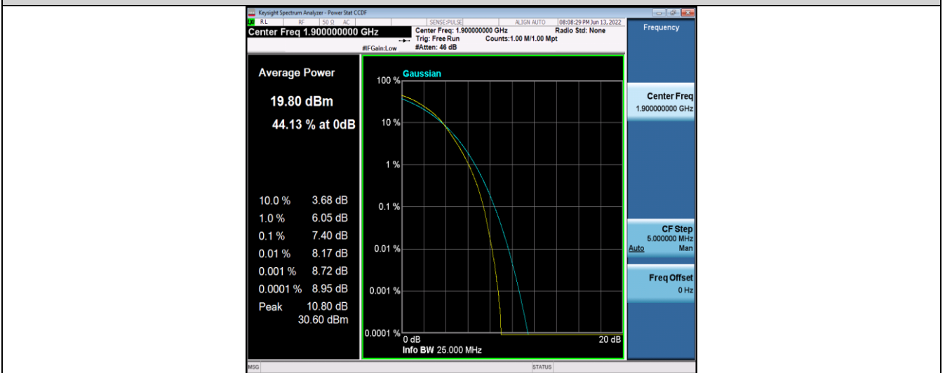
Band2-20MHz-16QAM-19100-100RB#0
