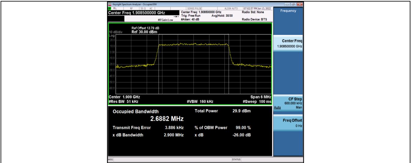
Band2-3MHz-16QAM-18615-15RB#0
