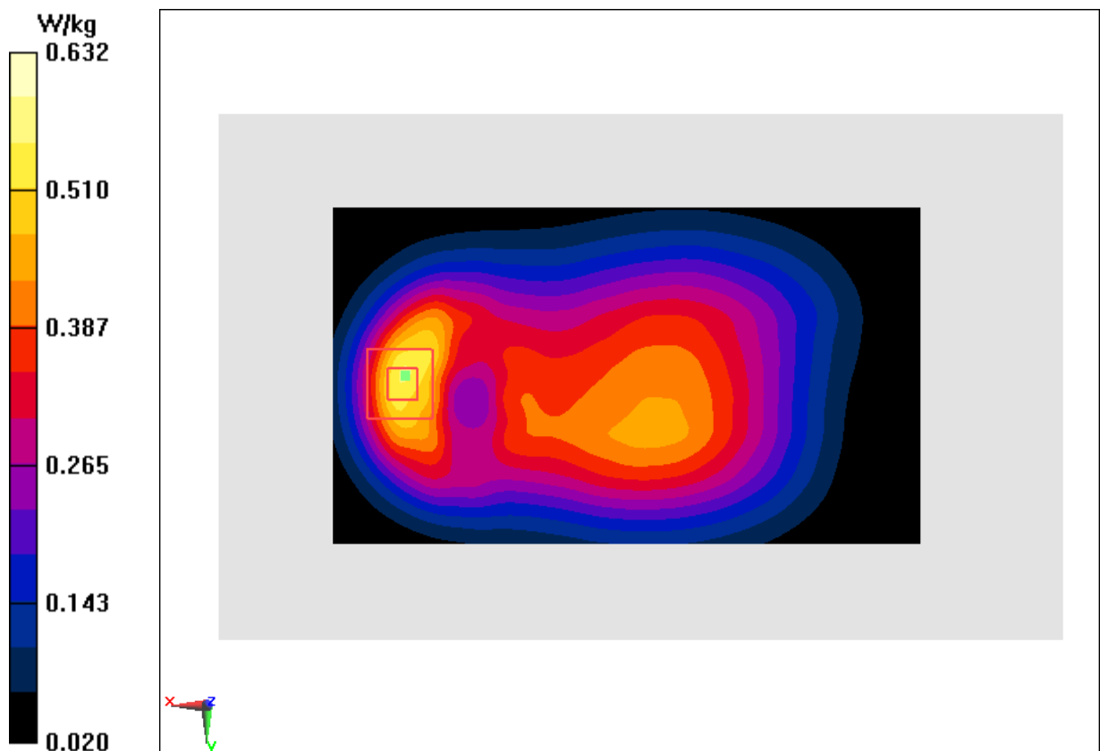
Fig.8LTE Band5
