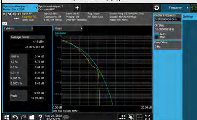
15MHz / 256QAM
