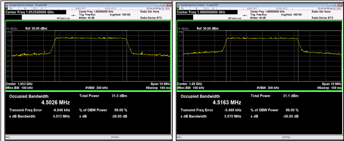
Band2-5MHz-QPSK-18625-25RB#0-PASS
