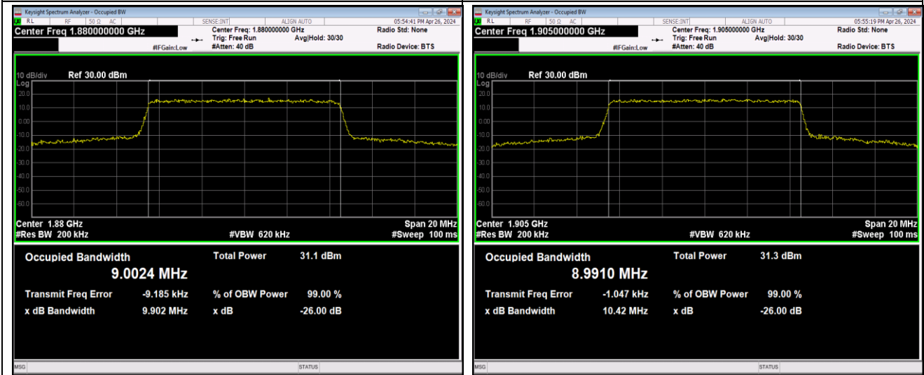
Band2-10MHz-QPSK-18900-50RB#0-PASS
