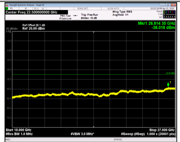
Band7_20MHz_QPSK_20850_1RB#0_18000~27000_18000~27000
