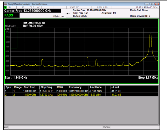
Band2_20MHz_QPSK_18700_1RB#99
