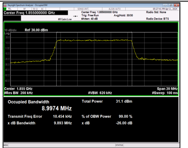
Band2-10MHz-QPSK-18650-50RB#0-PASS
