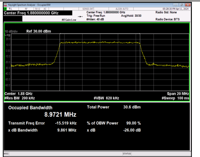
Band2-10MHz-16QAM-18900-50RB#0-PASS
