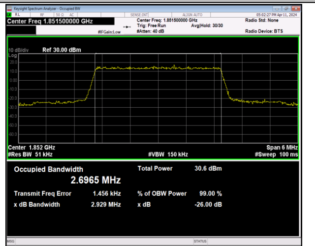
Band2-3MHz-QPSK-18615-15RB#0-PASS
