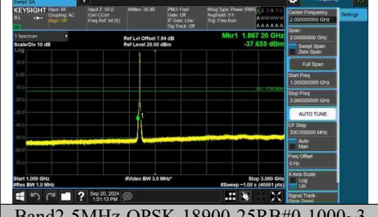
Band2-5MHz-QPSK-18900-25RB#0-1000~3 000-PASS
