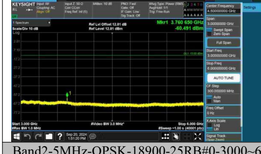
Band2-5MHz-QPSK-18900-25RB#0-3000~6 000-PASS
