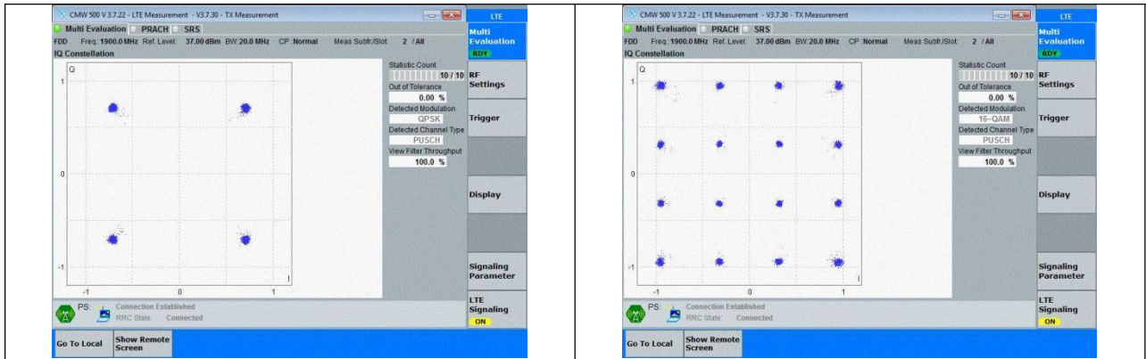
Band2-20MHz-QPSK-19100-100RB#0-PASS
