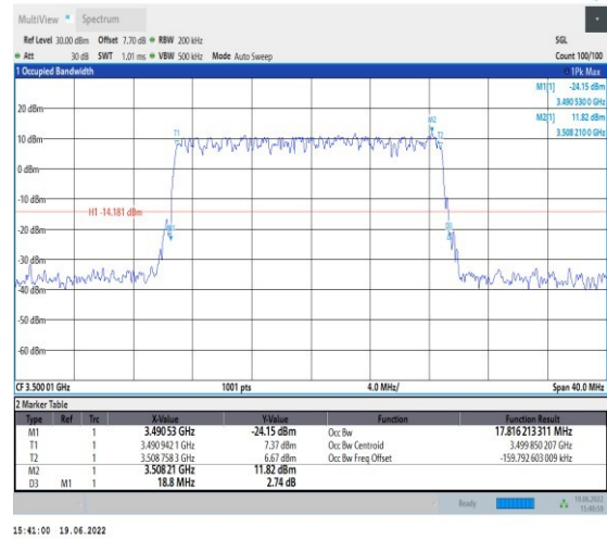
1-N78-3450-3550-PC2-30-20-M-5-DFT-256QAM-Out er_Full-50@0-Ant1-17.816-18.800-≤20-PASS
