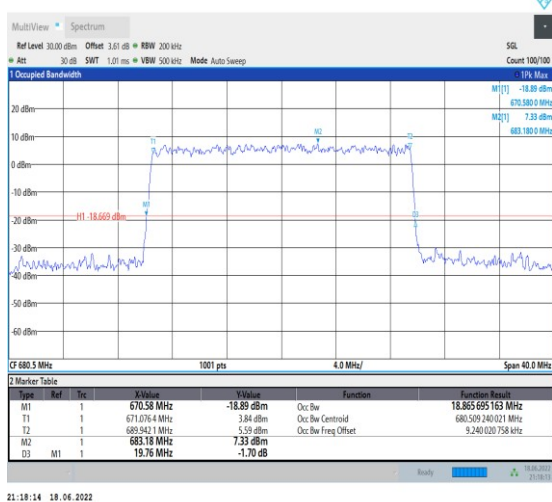
1-N71--15-20-M-9-CP-256QAM-Outer_Full-106@0-A nt1-18.866-19.760-≤20-PASS
