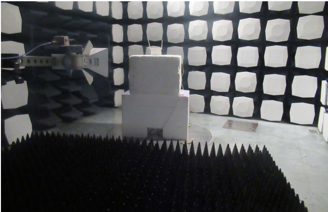
1GHz-18GHz
