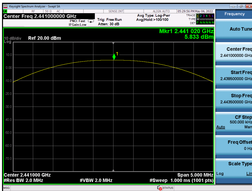
GFSK 2441MHz
