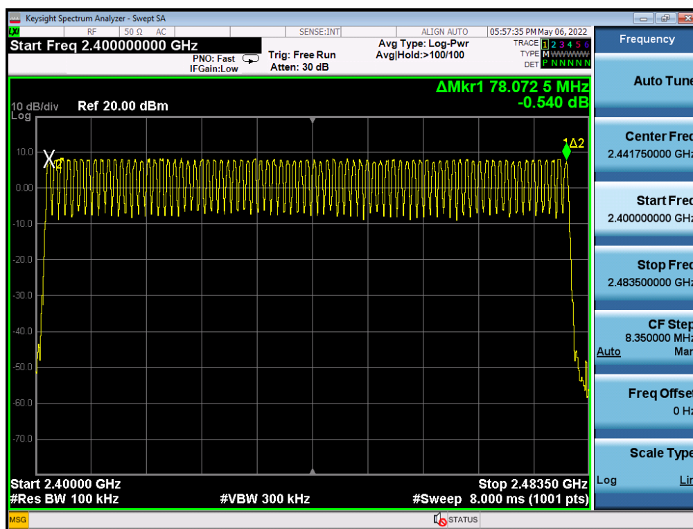
GFSK
