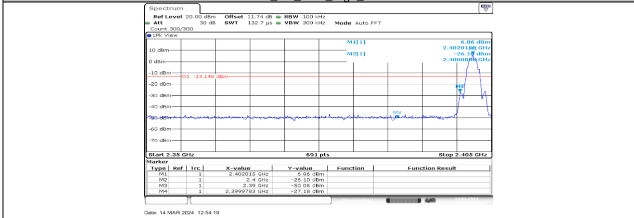
BLE_2M_Ant2_Low_2402
