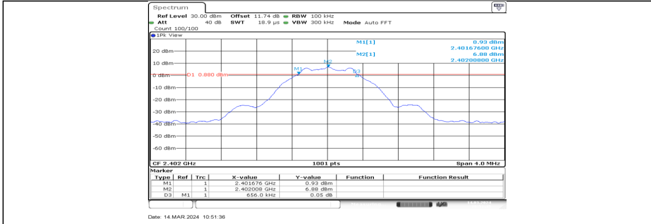
BLE_1M_Ant2_2402
