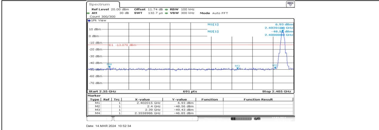
BLE_1M_Ant2_Low_2402
