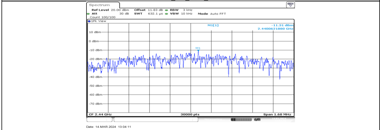
BLE_2M_Ant2_2440
