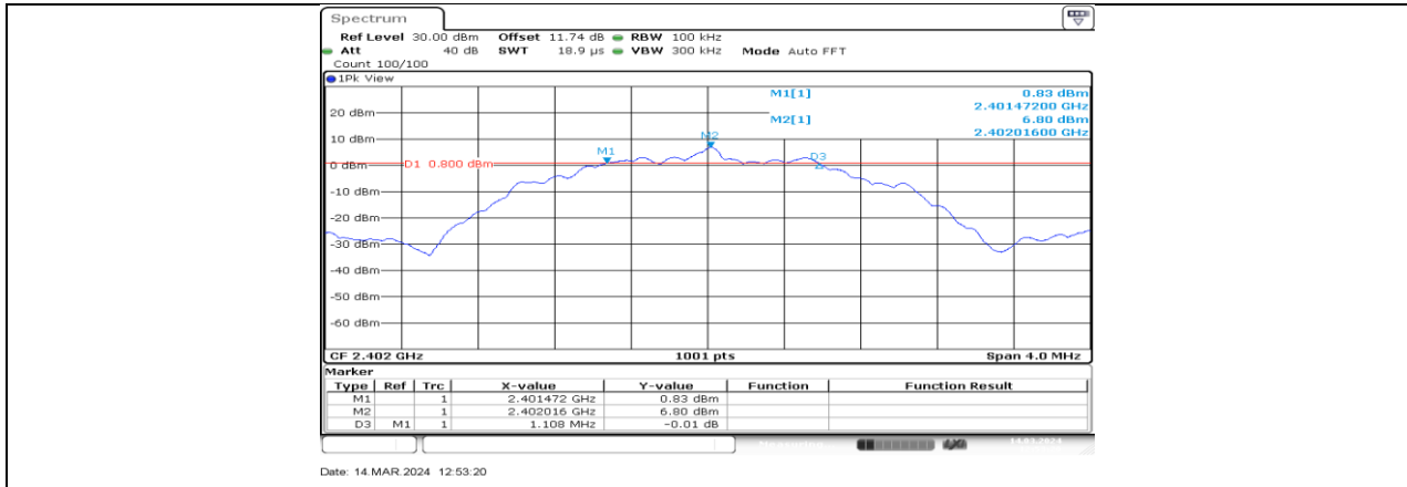
BLE_2M_Ant2_2402
