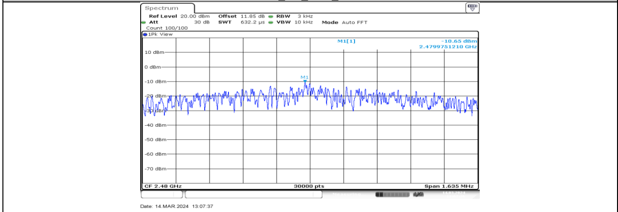
BLE_2M_Ant2_2480
