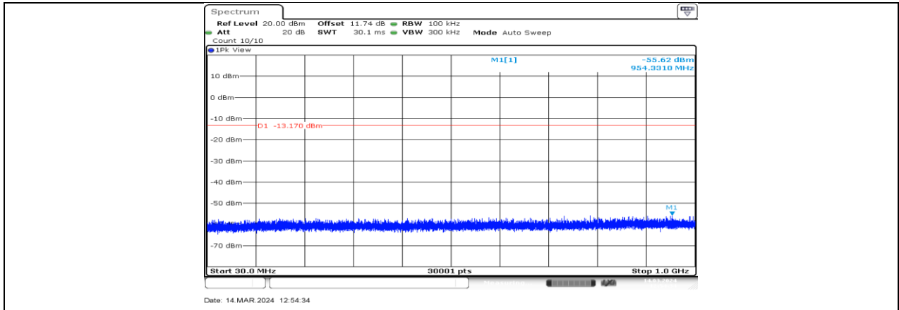
BLE_2M_Ant2_2402_30~1000
