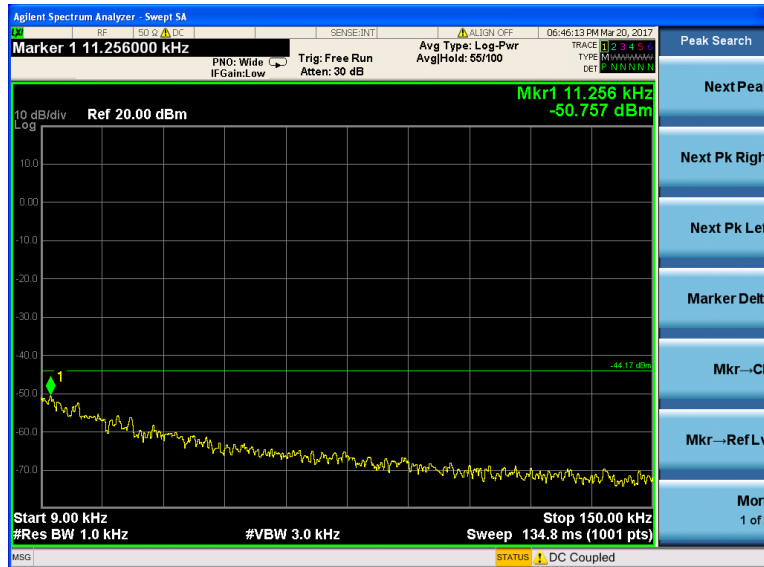
9KHz~150KHz
