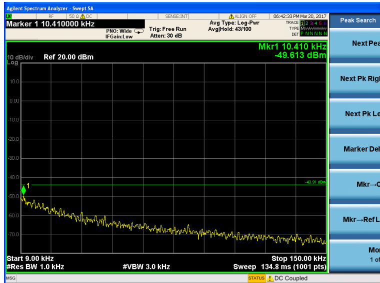
9KHz~150KHz
