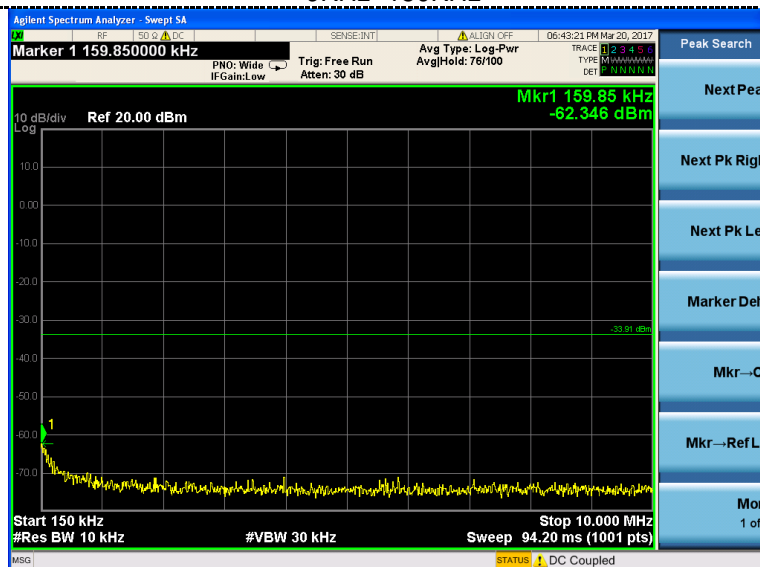
150KHz ~10MHz
