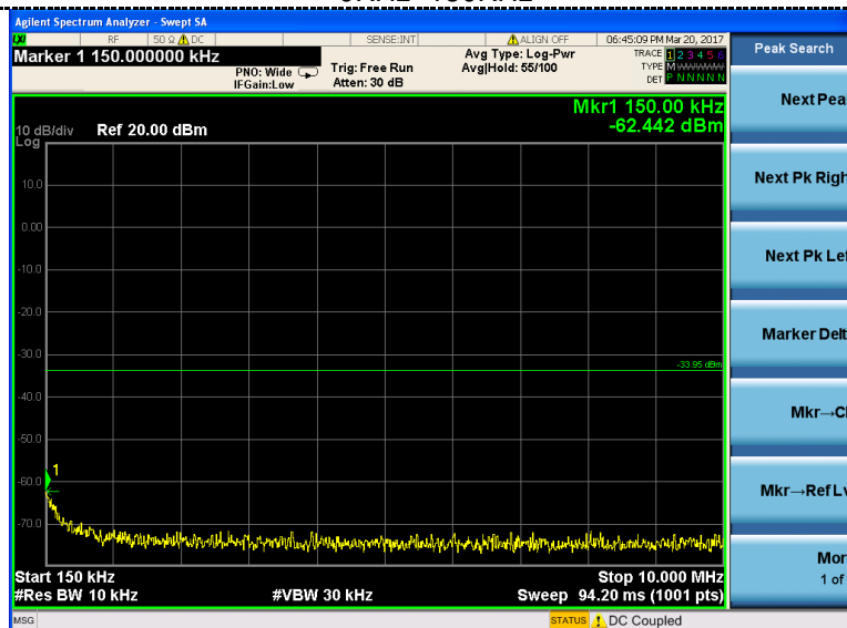
150KHz ~10MHz
