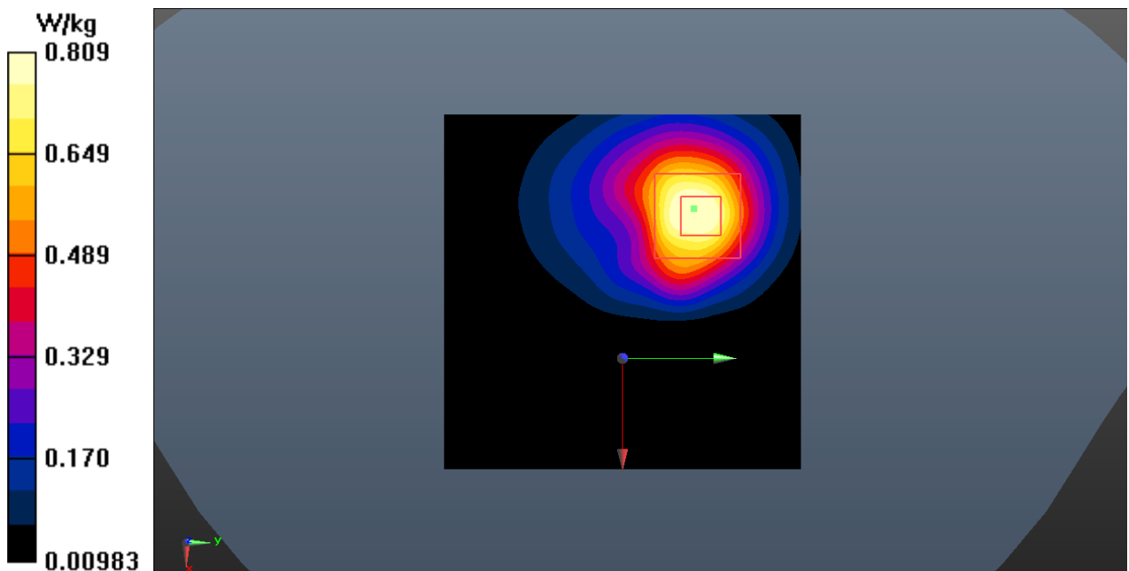
Fig.9 WCDMA 1700
