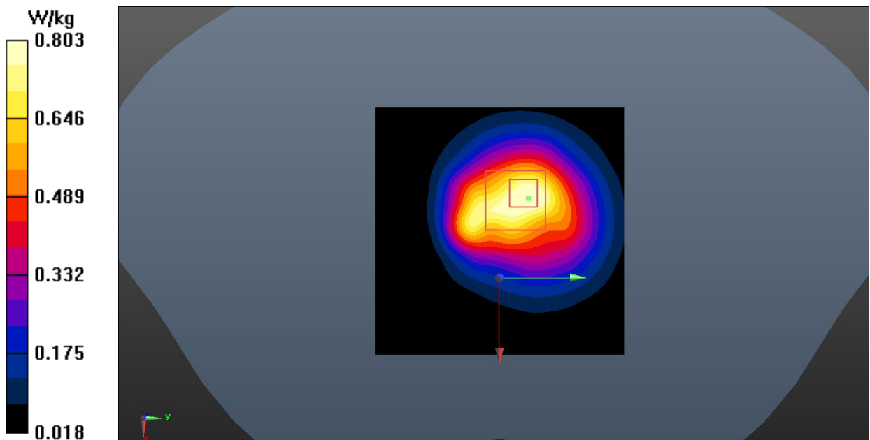
Fig.6 WCDMA 850
