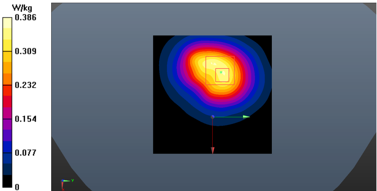
Fig.19 WLAN 2.4G
