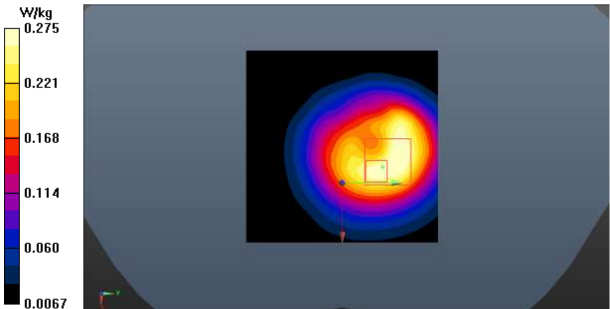
Fig.5 WCDMA 850
