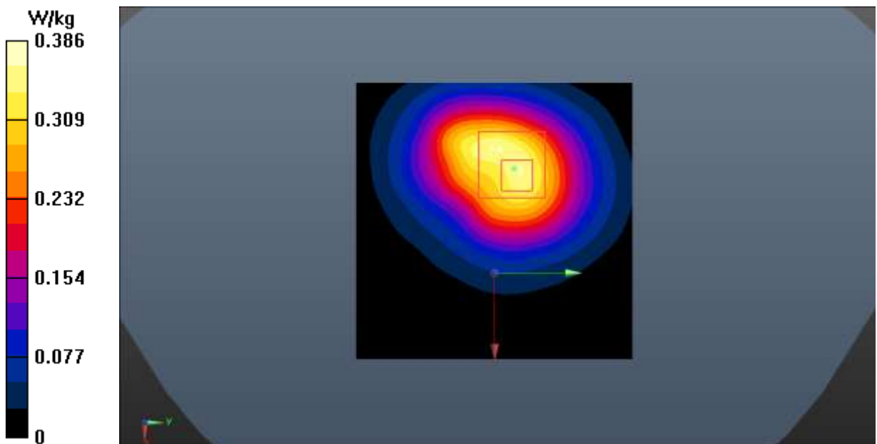
Fig.19 Wi-Fi 2.4G
