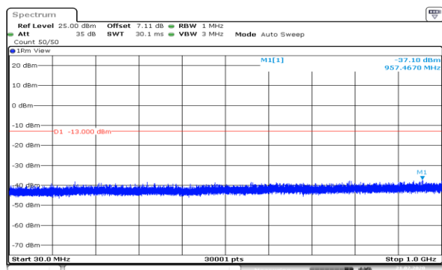
EGPRS_1900(8PSK)_Higher(30MHz-1GHz)
