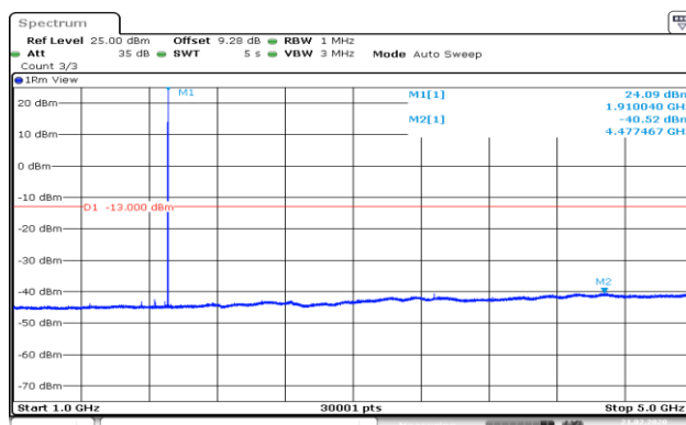
EGPRS_1900(8PSK)_Higher(1GHz-5GHz)
