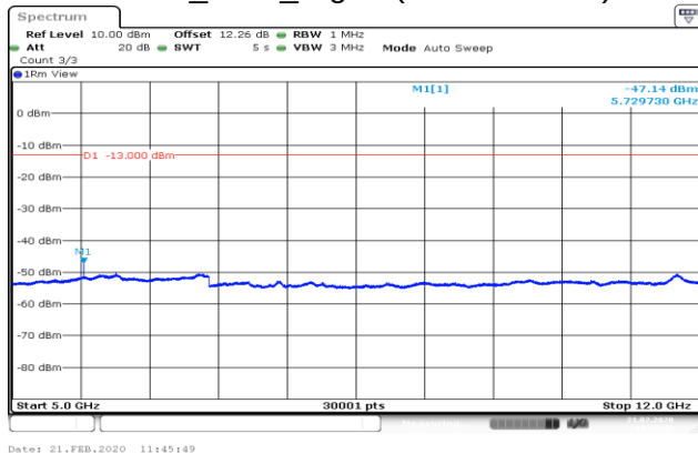
GPRS_1900_Higher(5GHz-12GHz)
