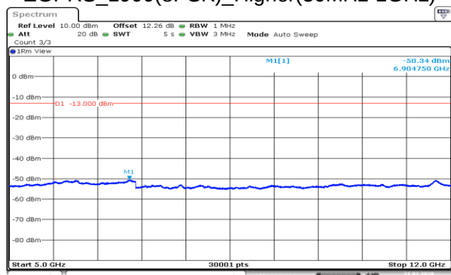
EGPRS_1900(8PSK)_Higher(5GHz-12GHz)
