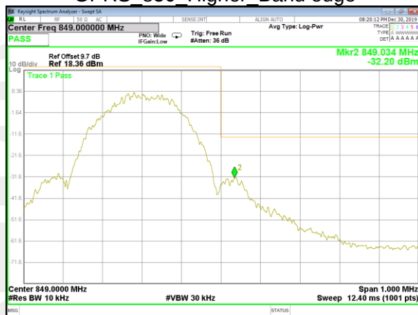
EGPRS_850(8PSK)_Higher_Band edge
