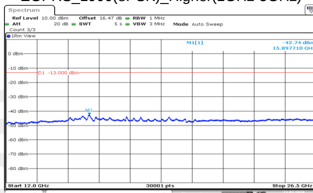
EGPRS_1900(8PSK)_Higher(12GHz-26.5GHz)
