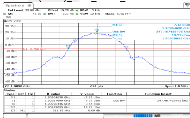
EGPRS(8PSK)_1900_Higher_26BW and 99%
