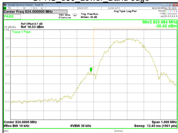
EGPRS_850(8PSK)_Lower_Band edge
